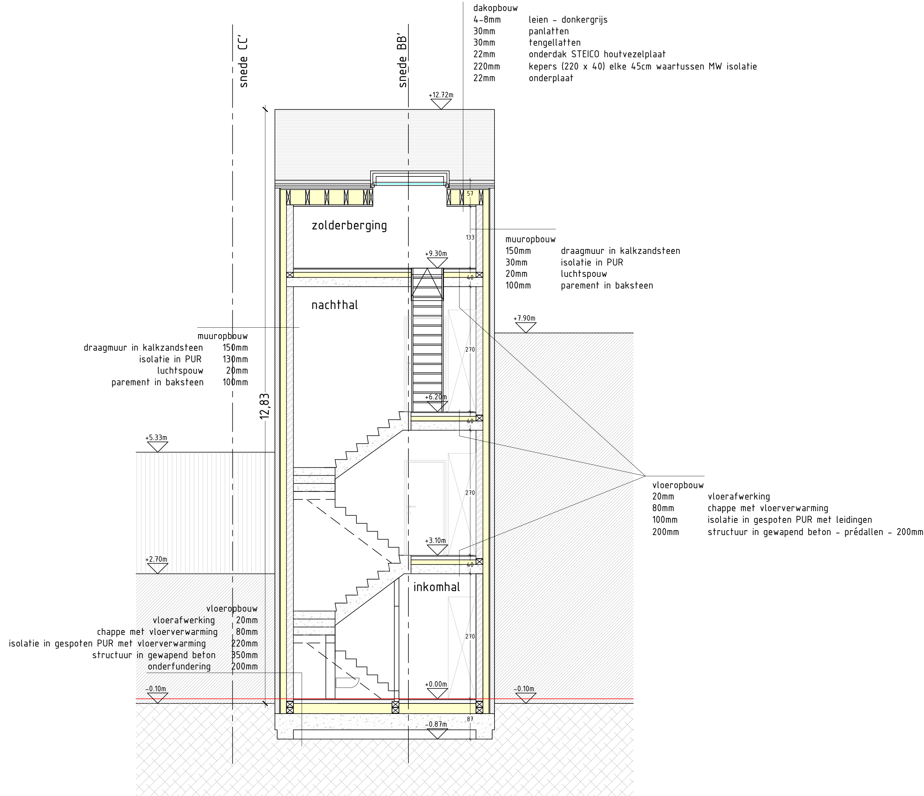
DOORSNEDE AA'
