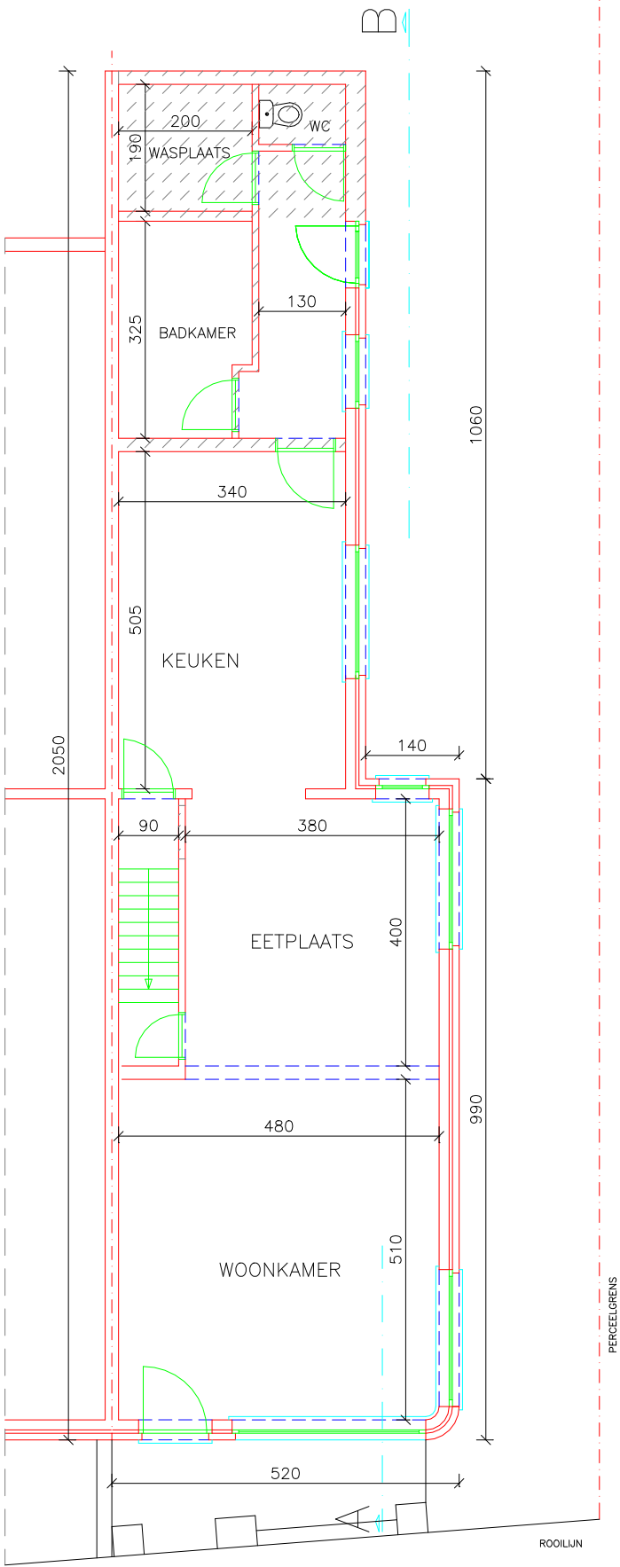
BA woning-P-B-1-gelijkvloers
