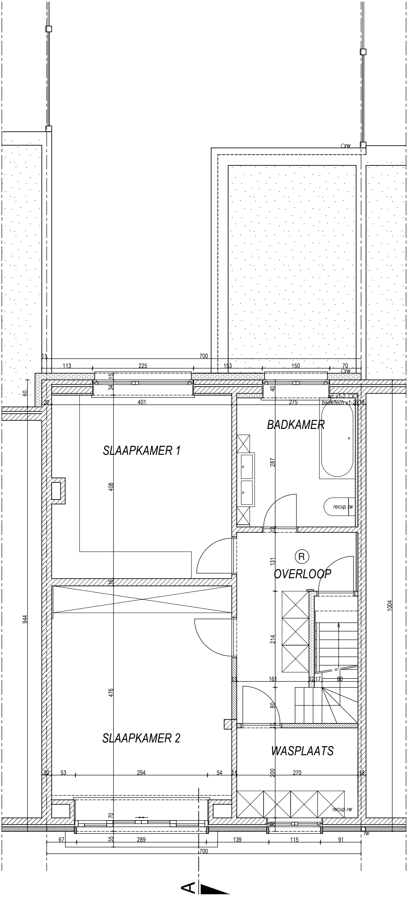
PLAN VERDIEPING 1 NIEUWE TOESTAND
