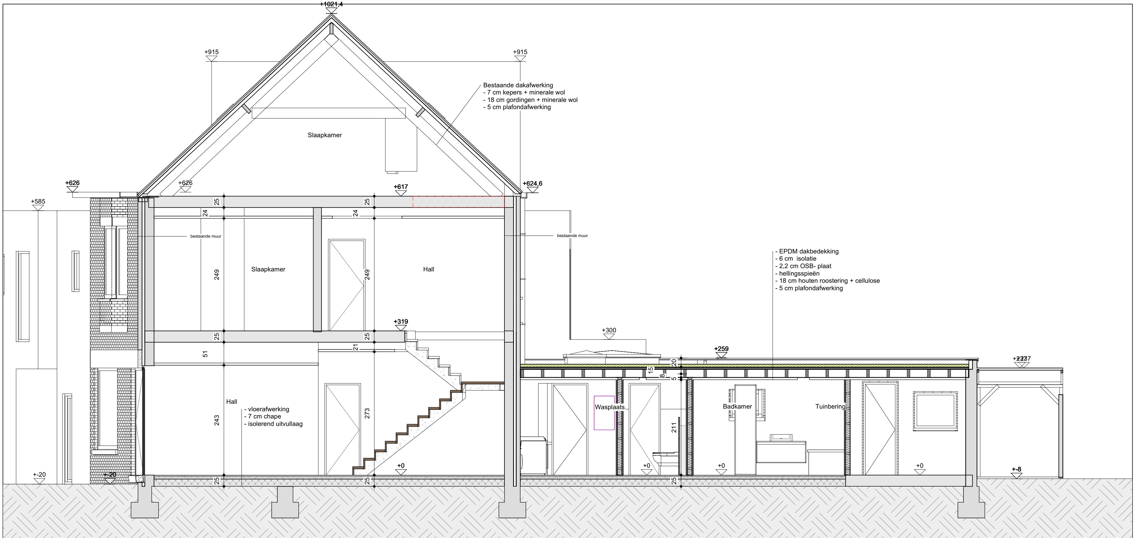
Langsdoorsnede A-A nieuwe toestand
