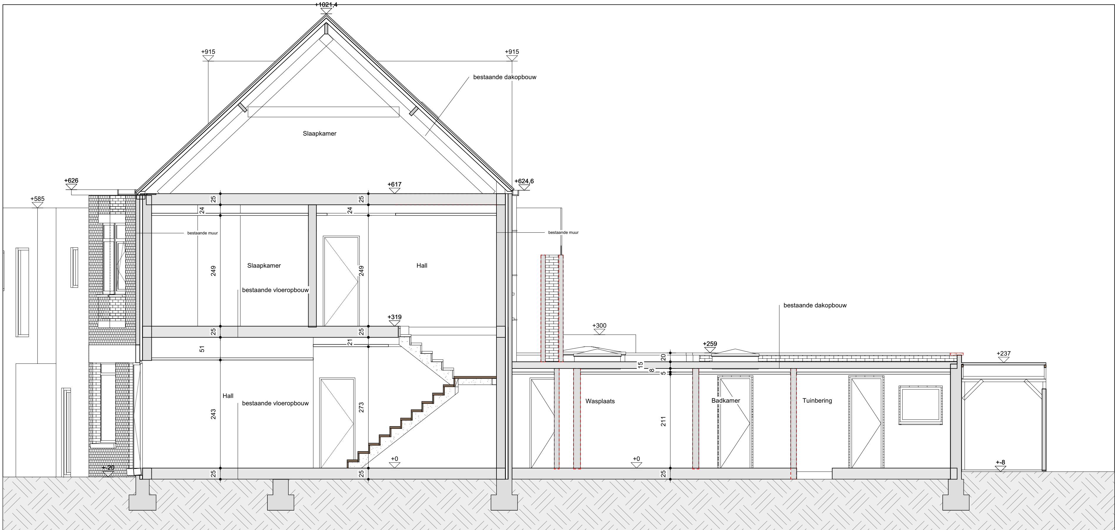
Langsdoorsnede A-A bestaande toestand
