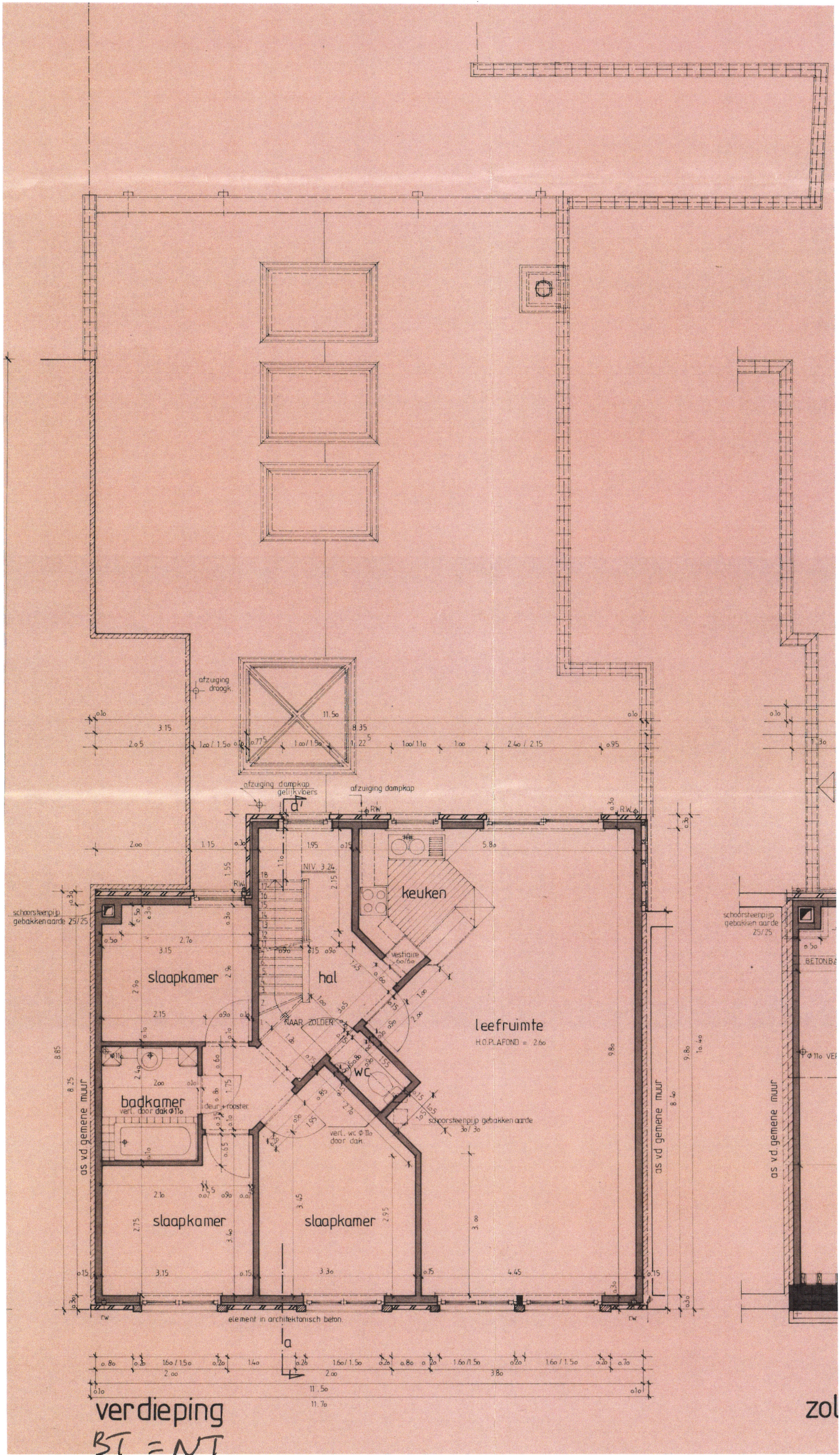
BA_Brugsesteenweg_65_P_BN_grondplan verdieping bestaande en nieuwe toestand
