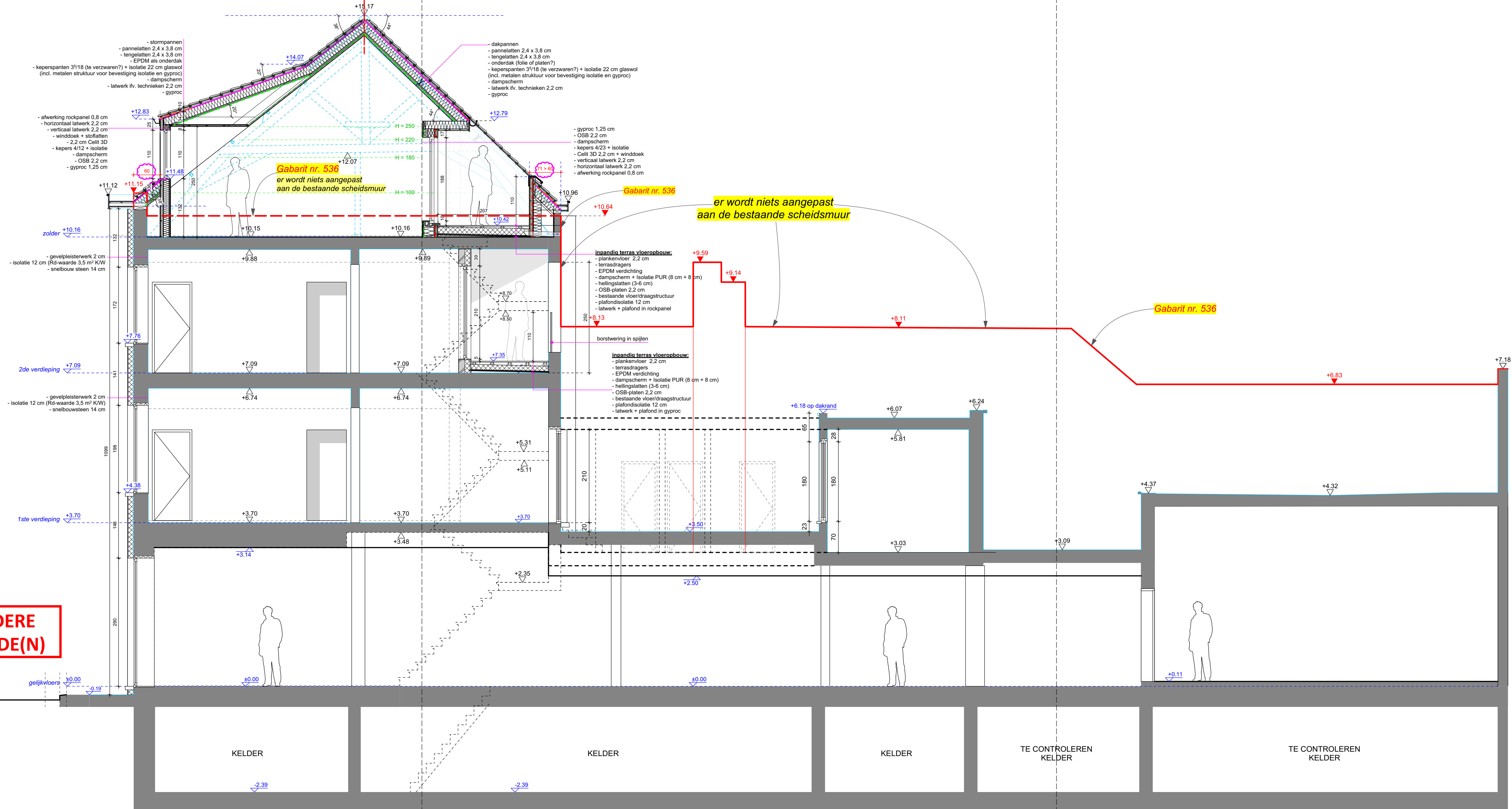
LANGSE SNEDE D-D' 1/50
