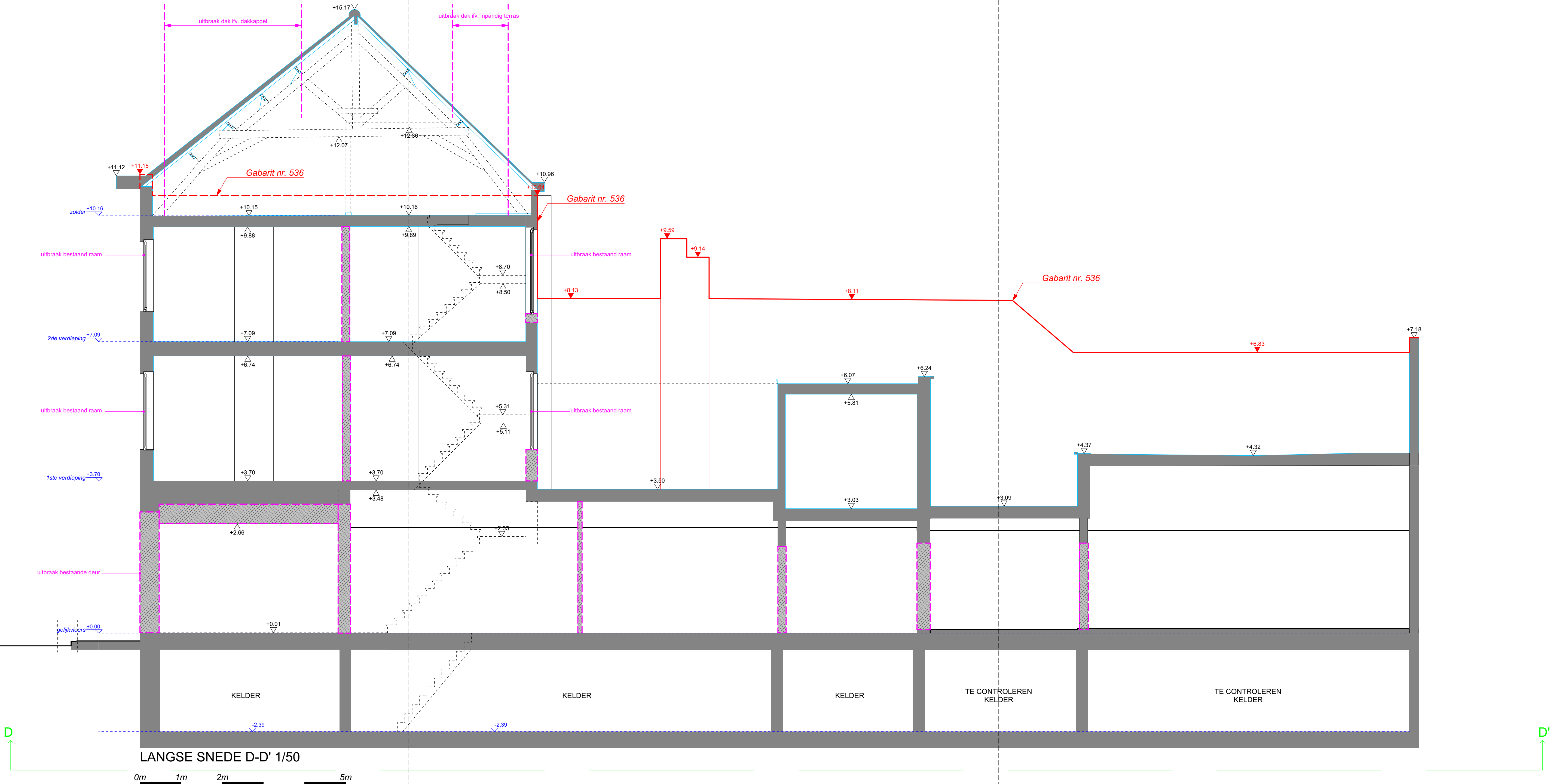
Doorsnede DD' : bestaande toestand
