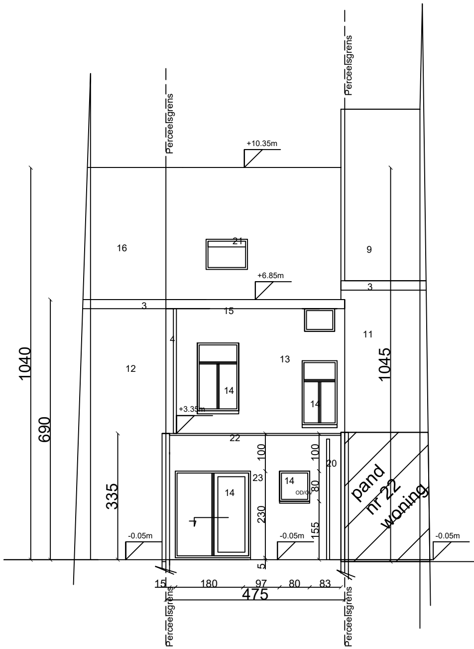
Achtergevel 1/100 NIEUWE TOESTAND
