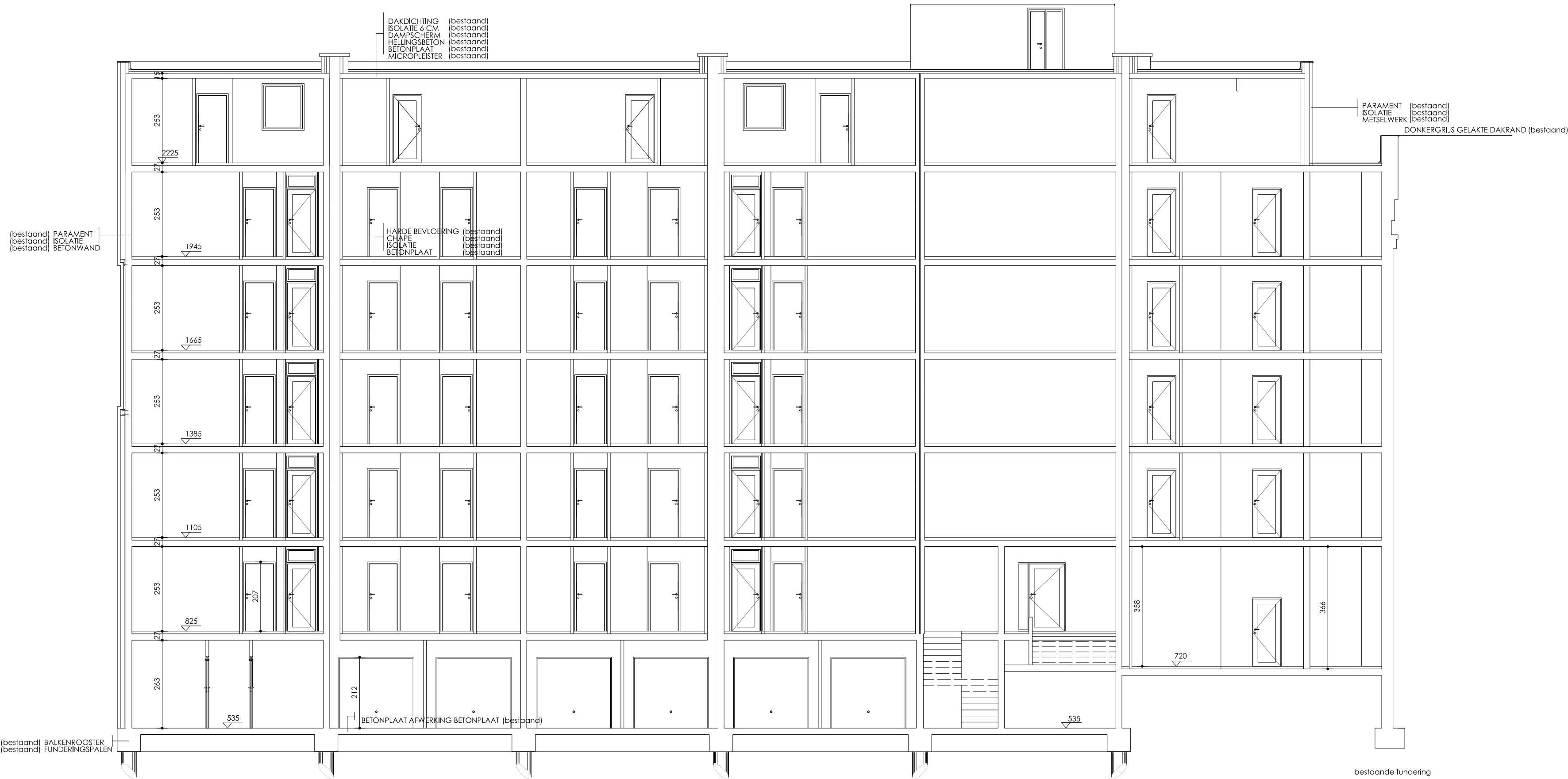
BLOK 205 DOORSNEDE A-A
