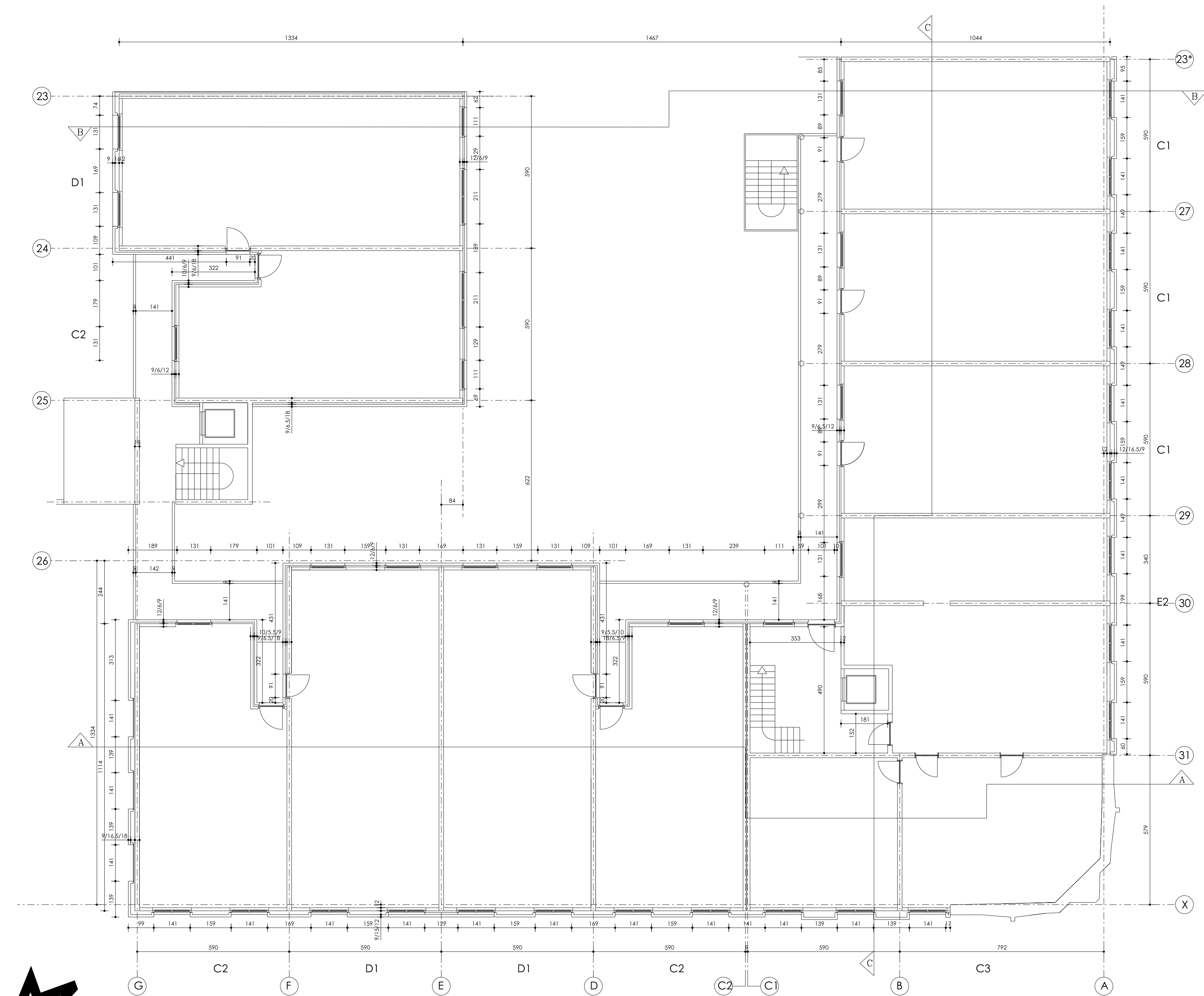
Blok 205 - Eerste verdieping
