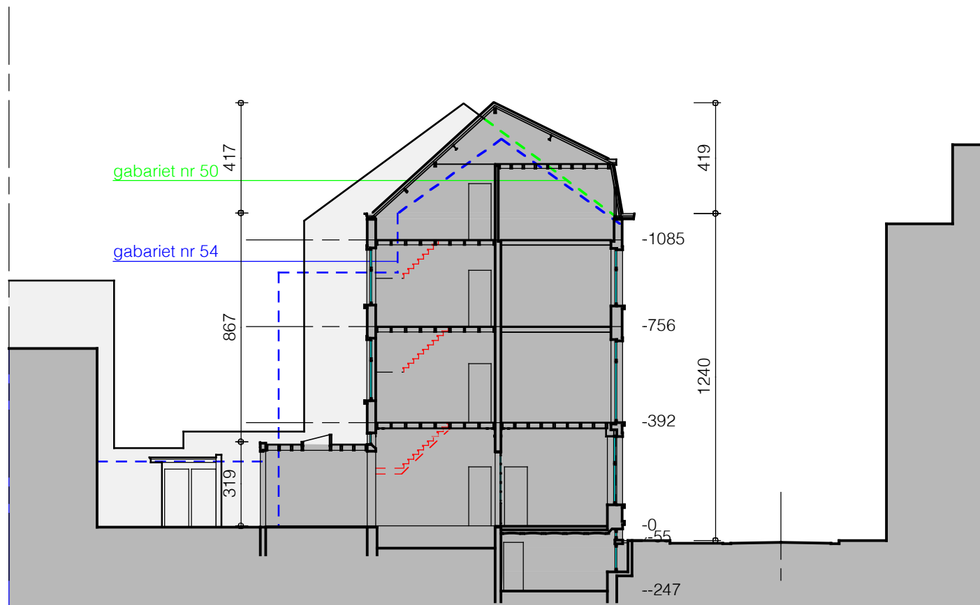
terreinprofiel 1 - bestaande toestand
