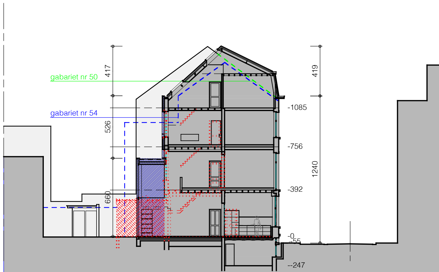
terreinprofiel 1 - nieuwe toestand
