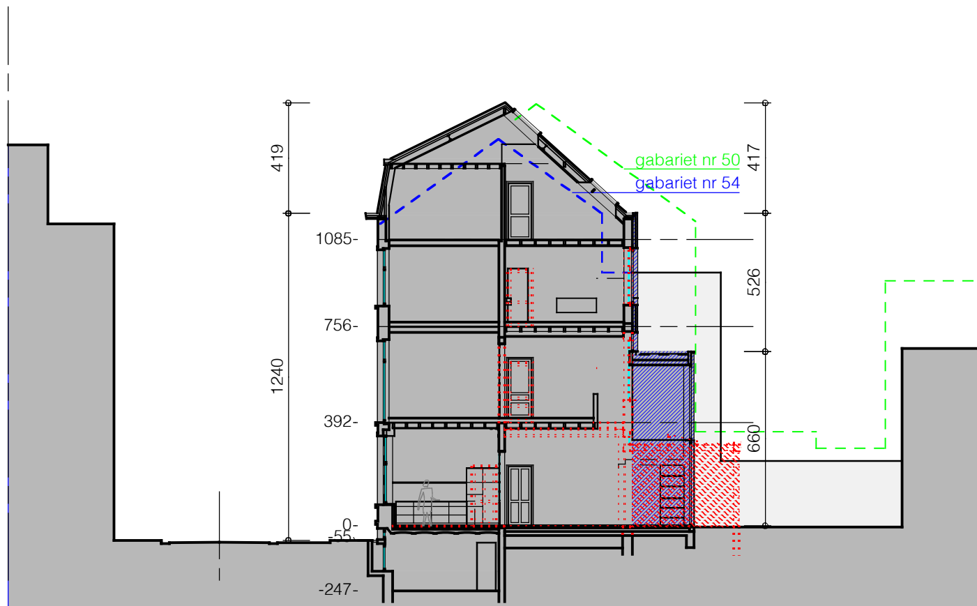
terreinprofiel 2 - nieuwe toestand
