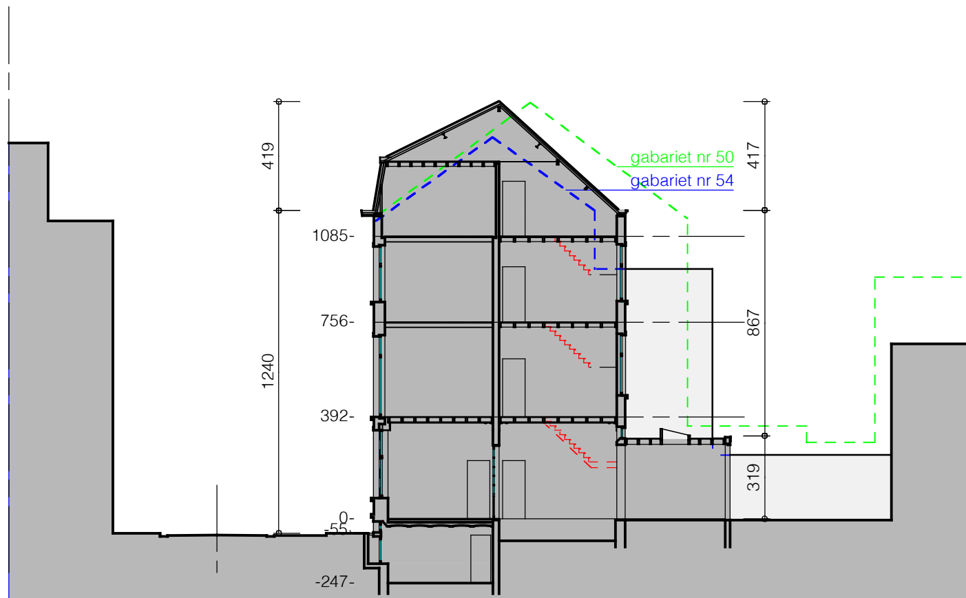
terreinprofiel 2 - bestaande toestand
