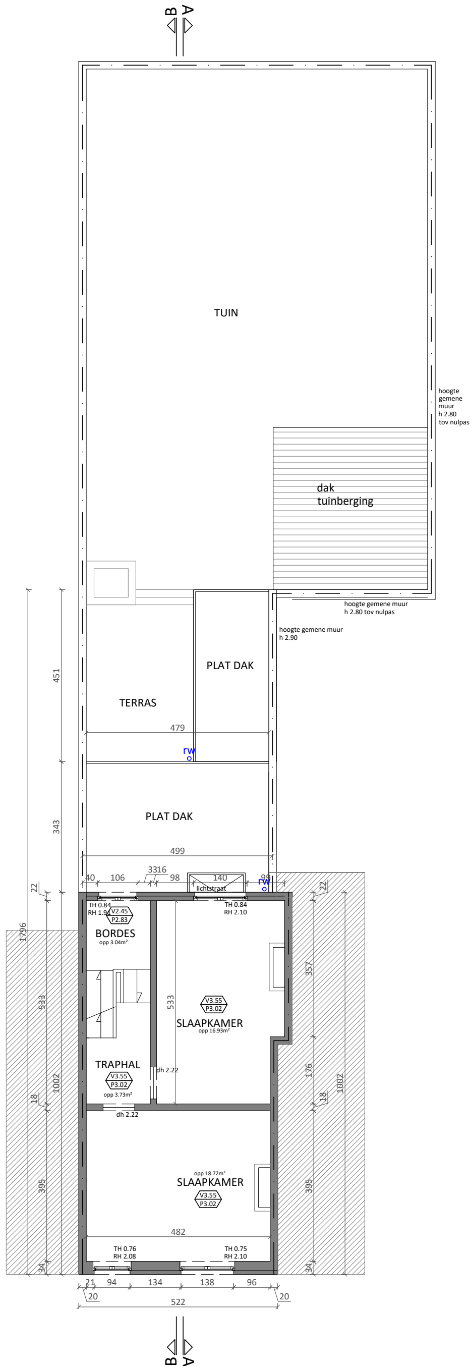
BESTAANDE TOESTAND EERSTE VERDIEPING 1-100
