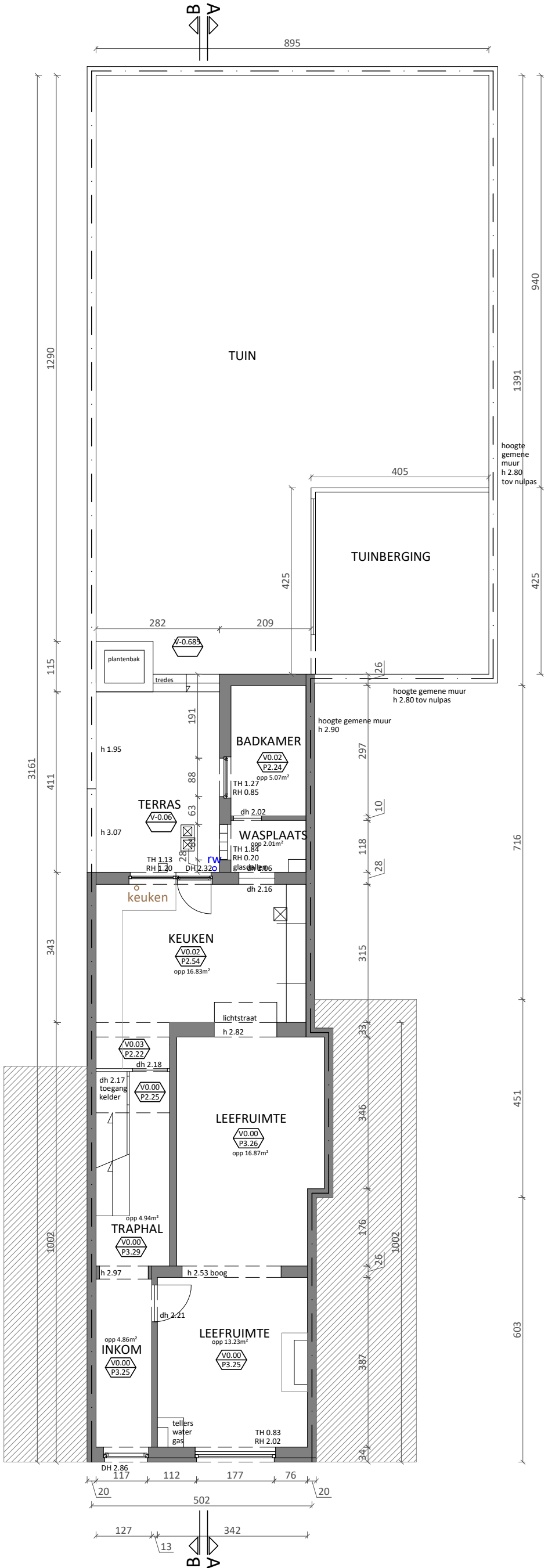
BESTAANDE TOESTAND GELIJKVLOERS 1-100
