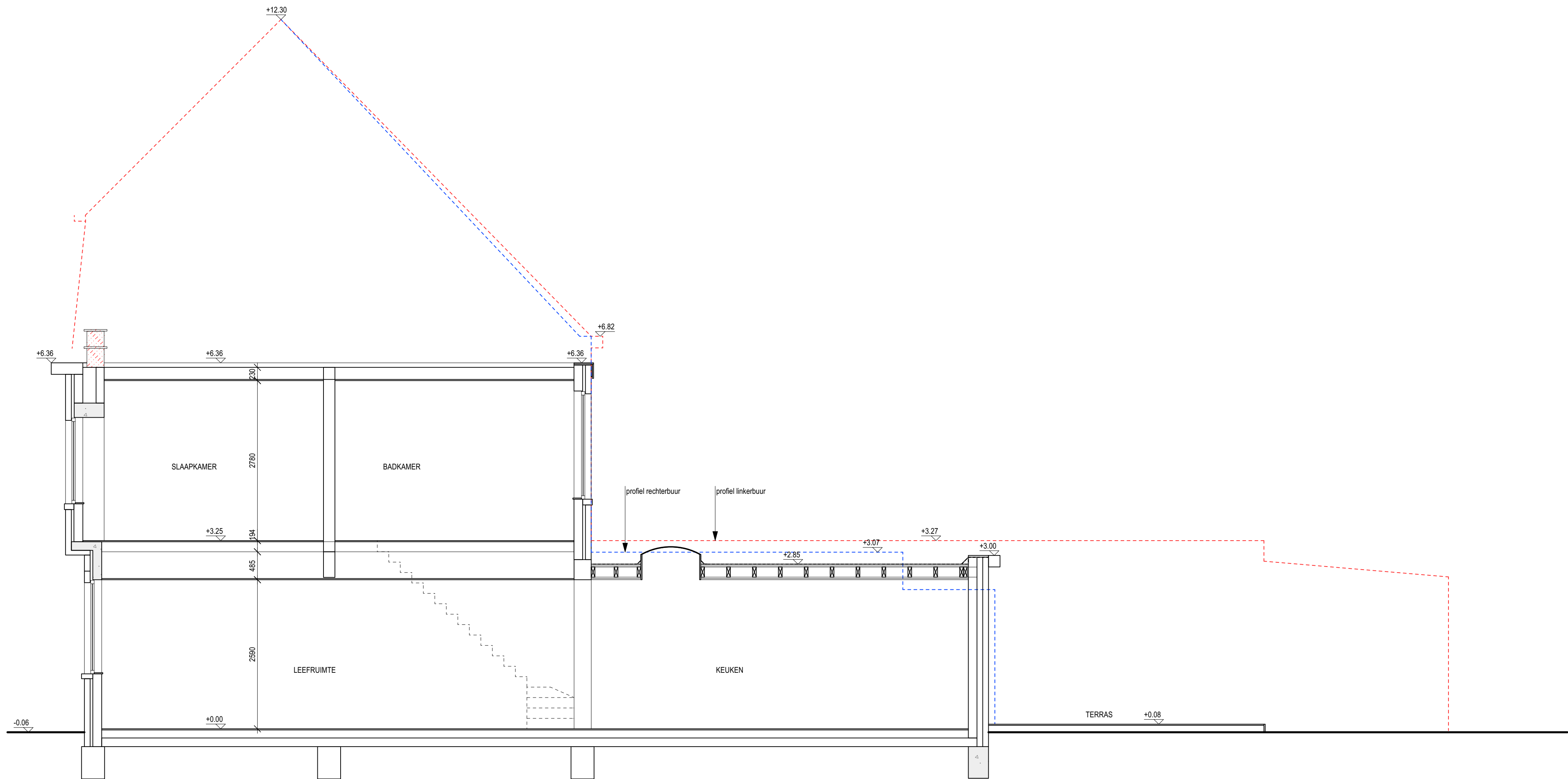
SNEDE BESTAANDE TOESTAND 1/50
