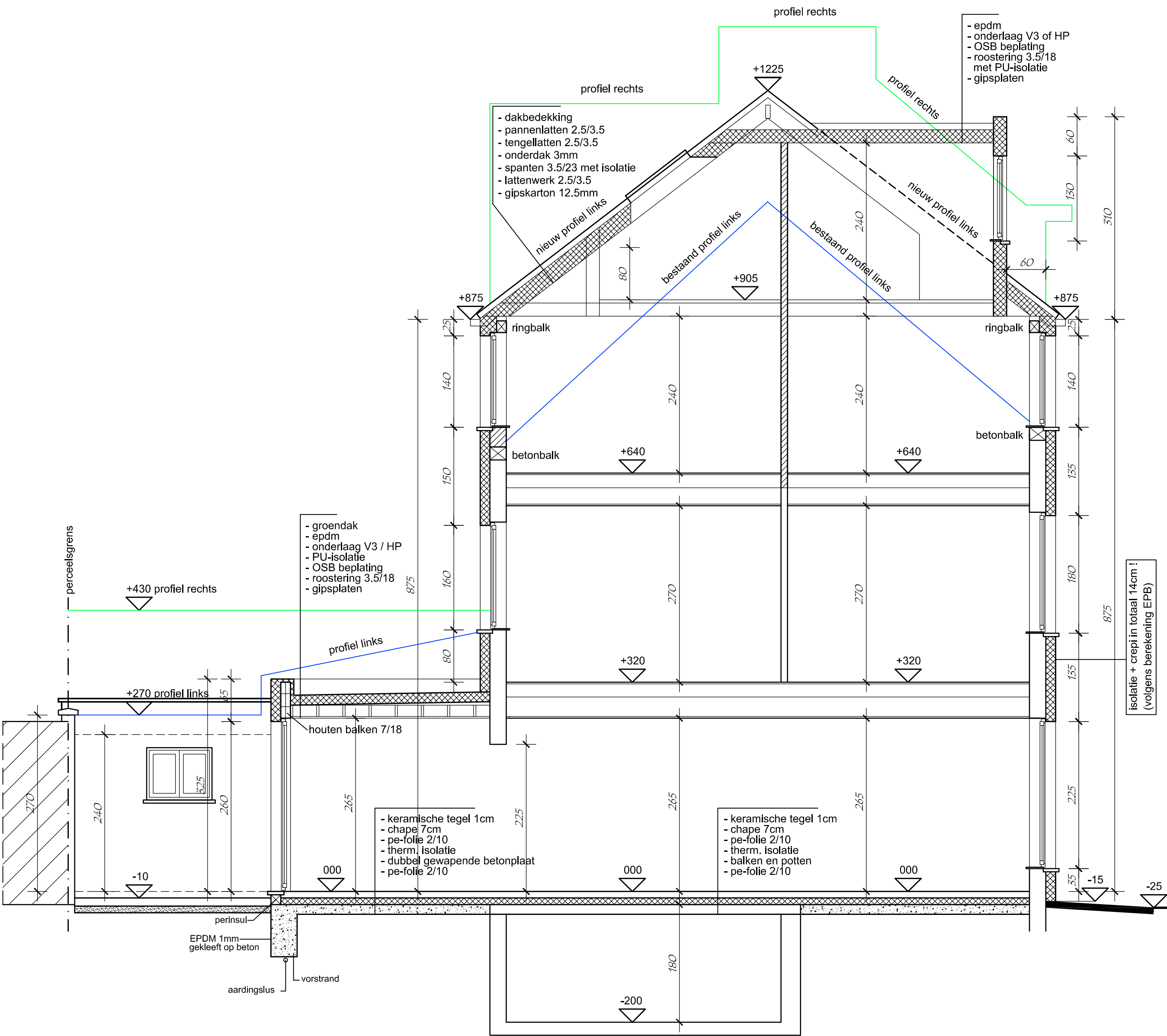
DOORSNEDE - TERREINPROFIEL 1/50
