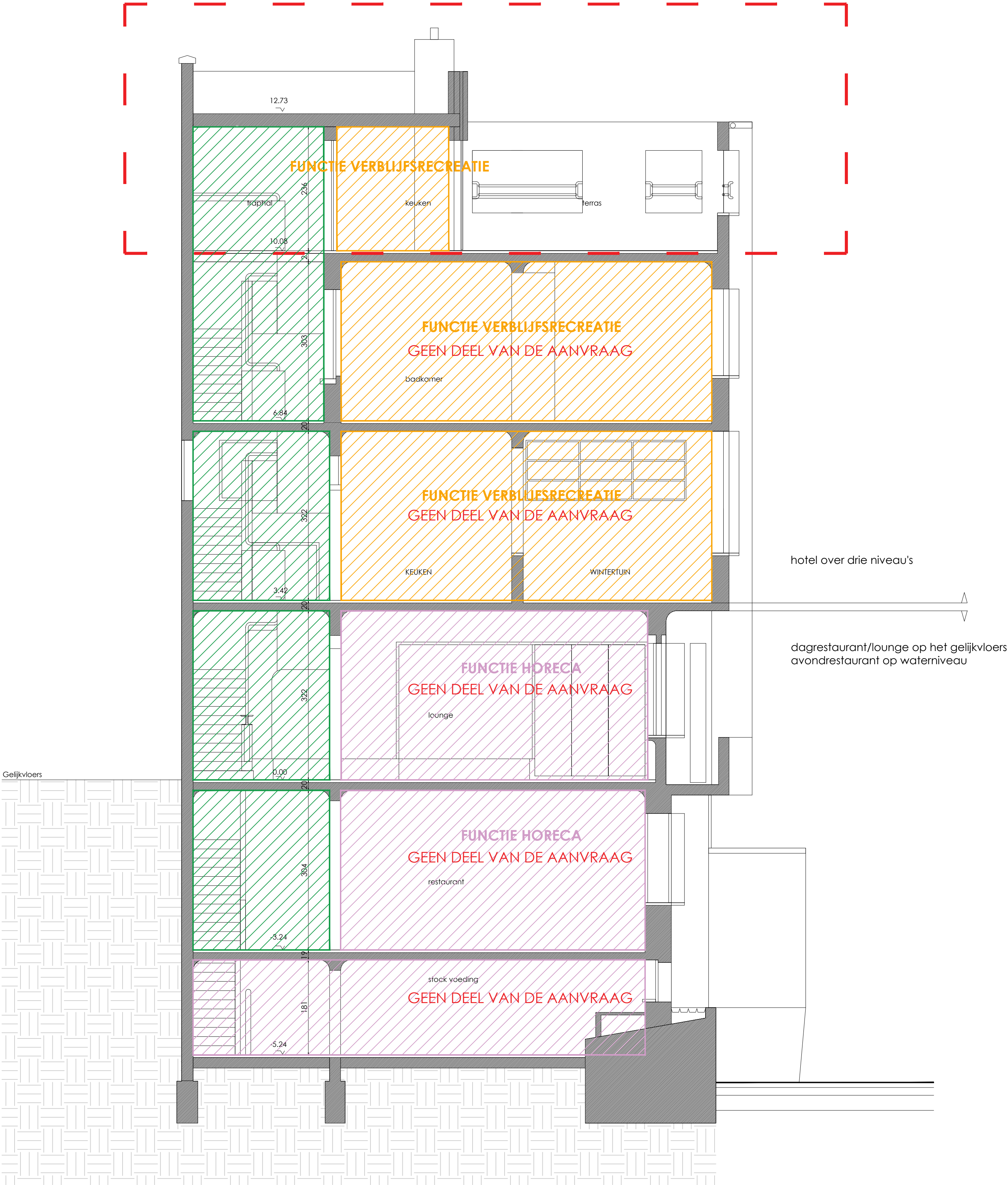
DOORSNEDE A-A'
