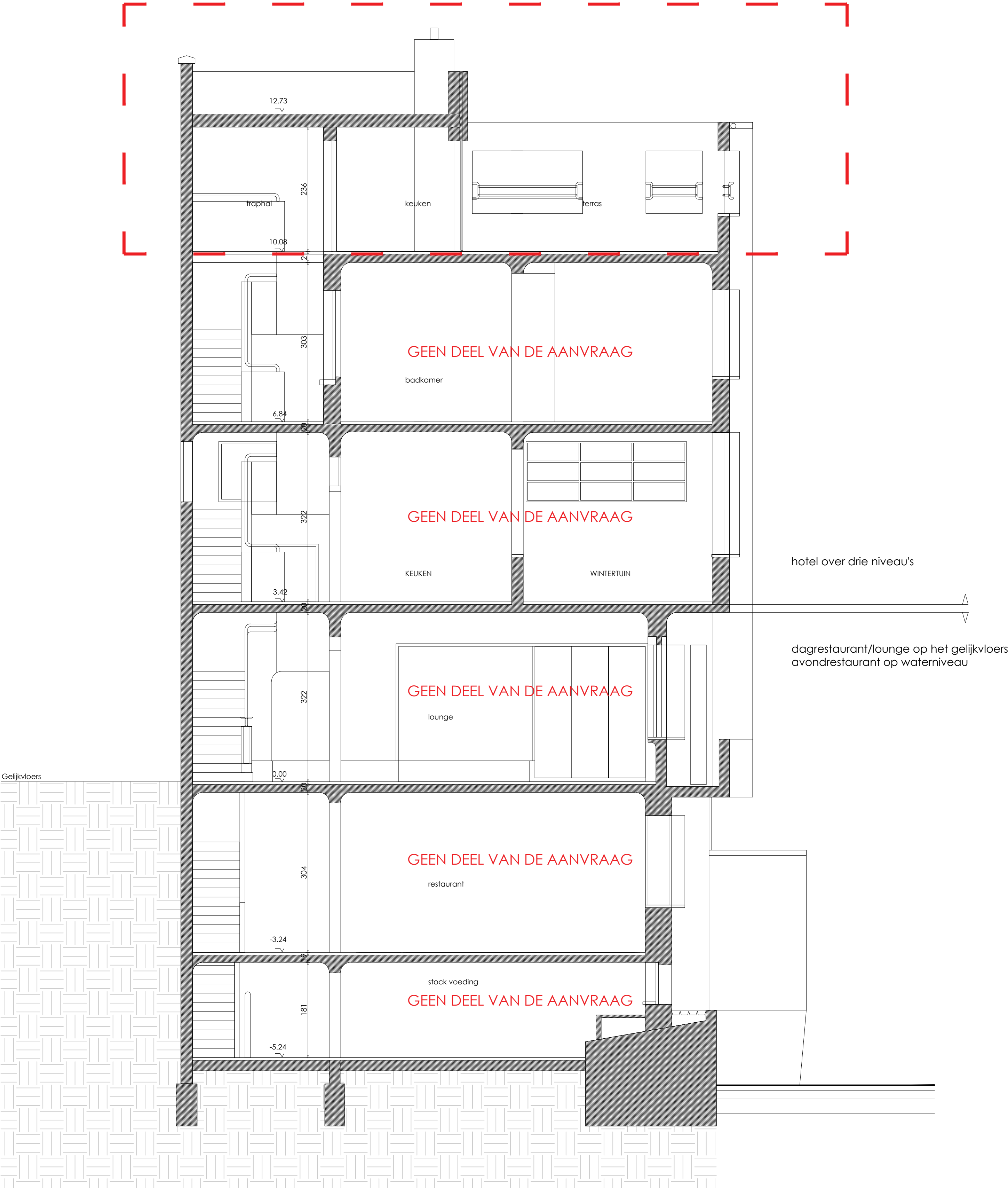
DOORSNEDE A-A'
