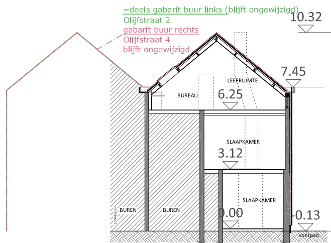
NIEUWE TOESTAND TERREINPROFIEL B-B 1-200
