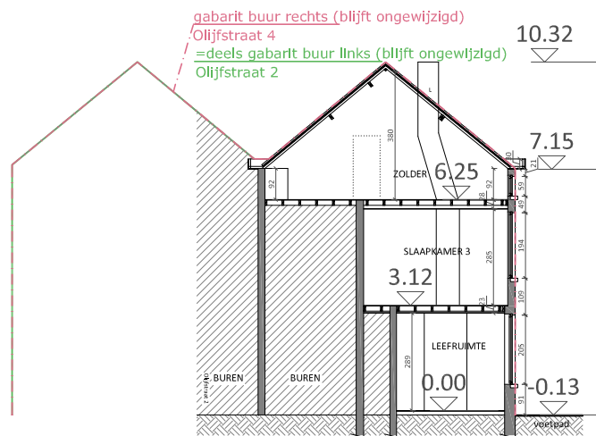
BESTAANDE TOESTAND TERREINPROFIEL B-B 1-100
