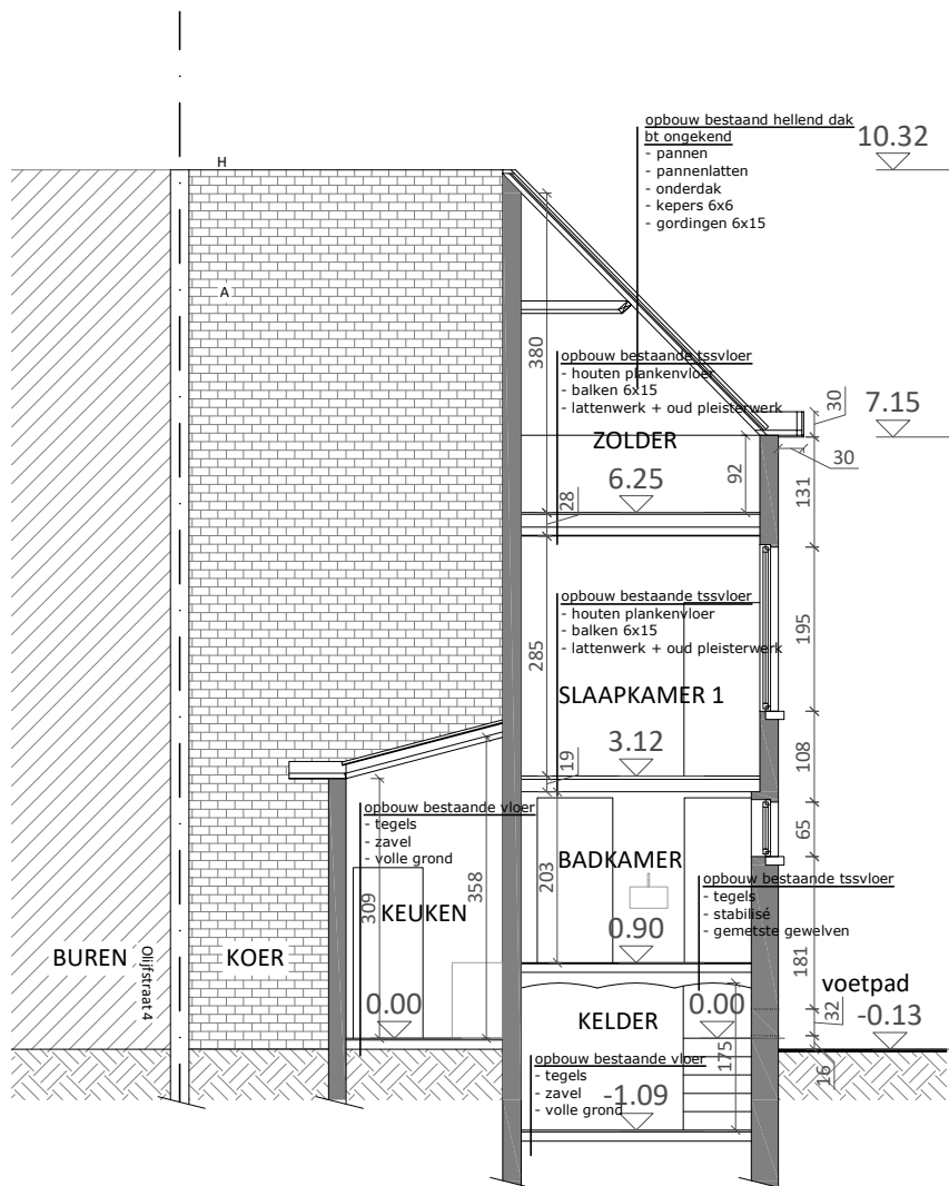
BESTAANDE TOESTAND SNEDE D-D 1-100 (=achtergevel)
