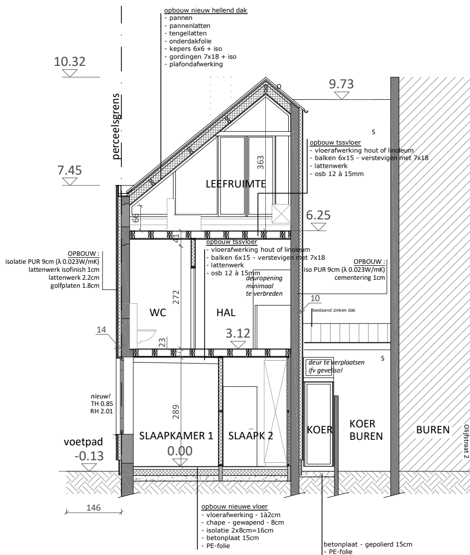
NIEUWE TOESTAND SNEDE A-A 1-100 (=achtergevel)
