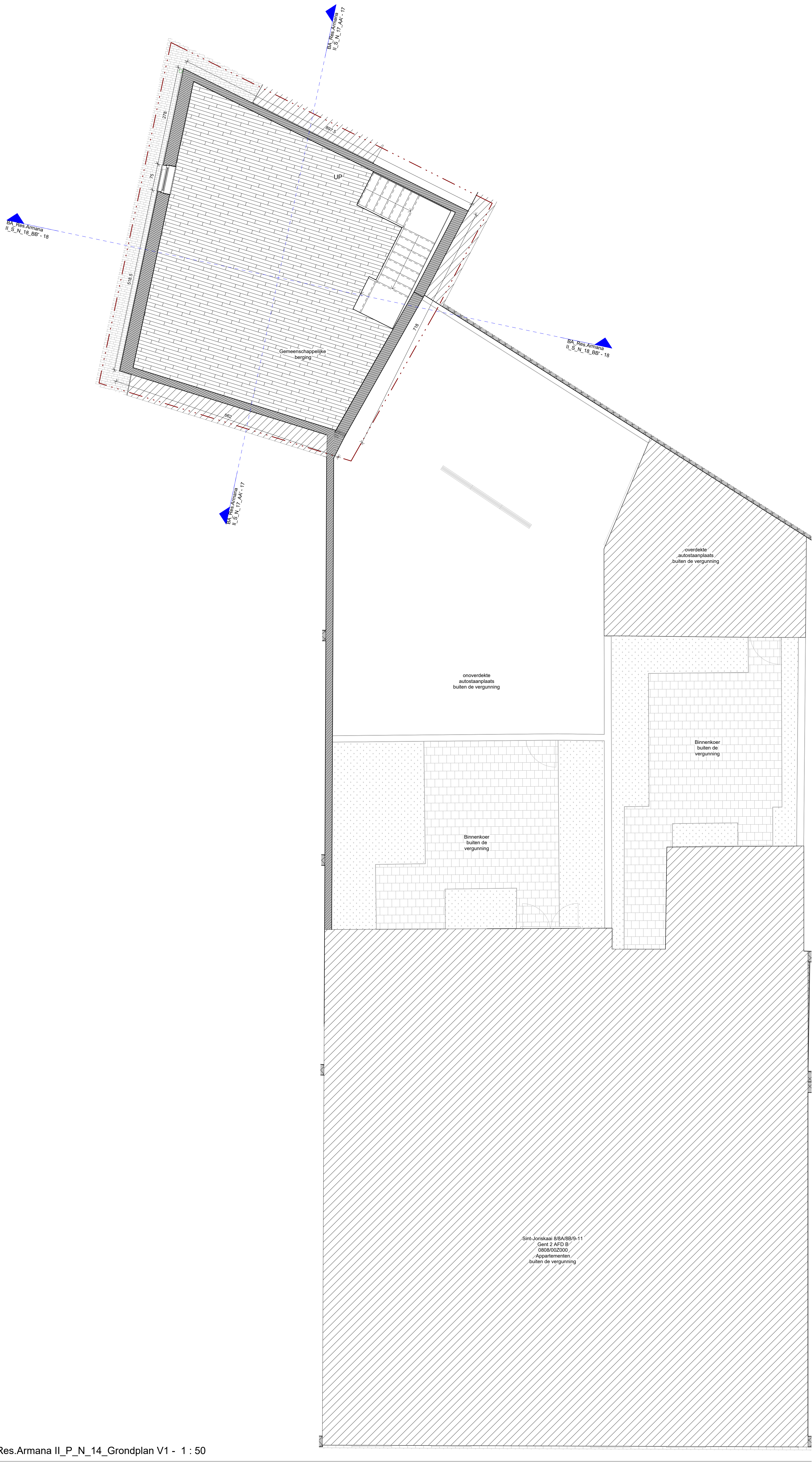
BA_Res.Armana II_P_N_14_Grondplan V1 - 1 : 50
