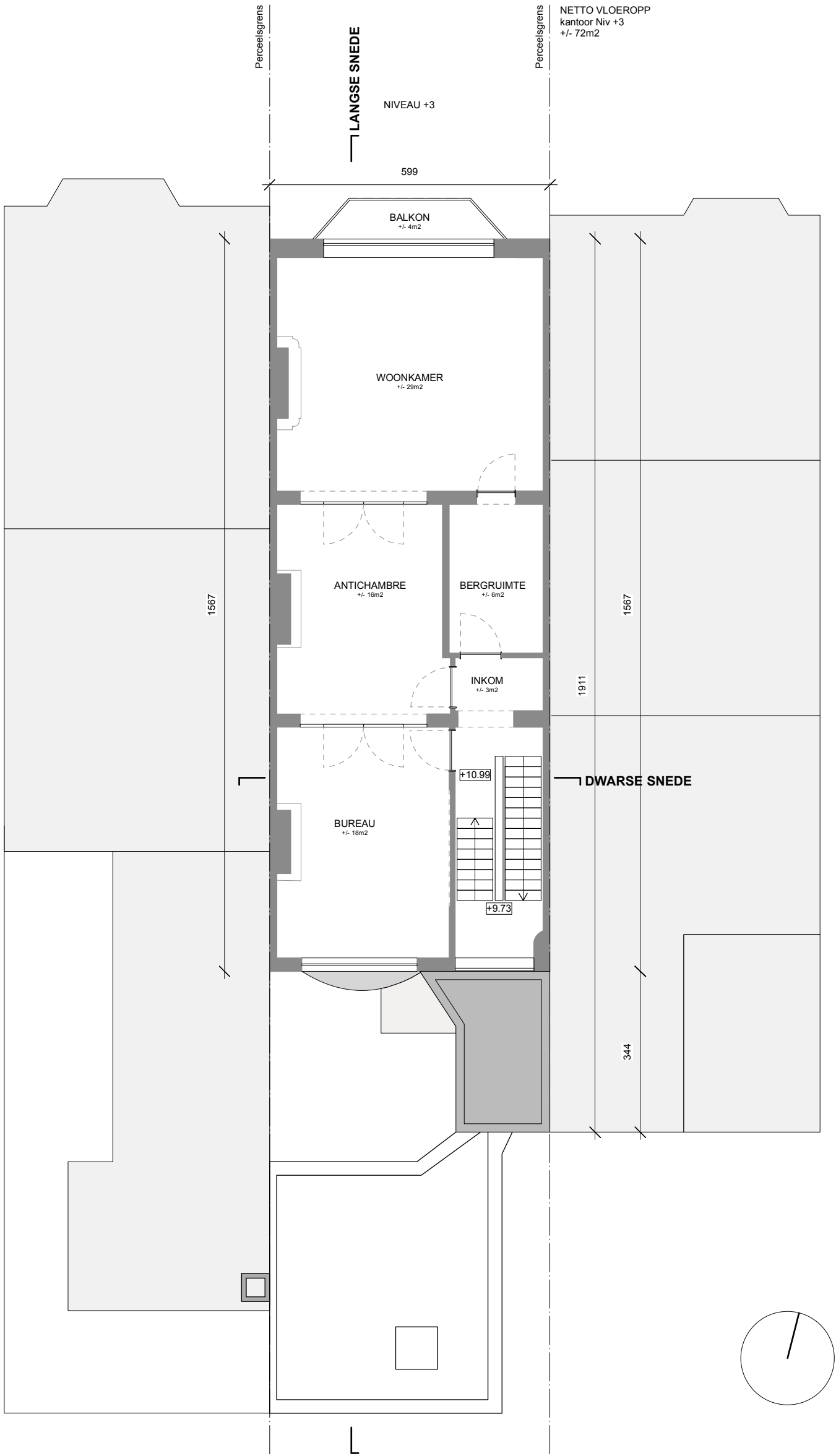
PLAN NIV+3 BESTAANDE TOESTAND schaal 1/100
