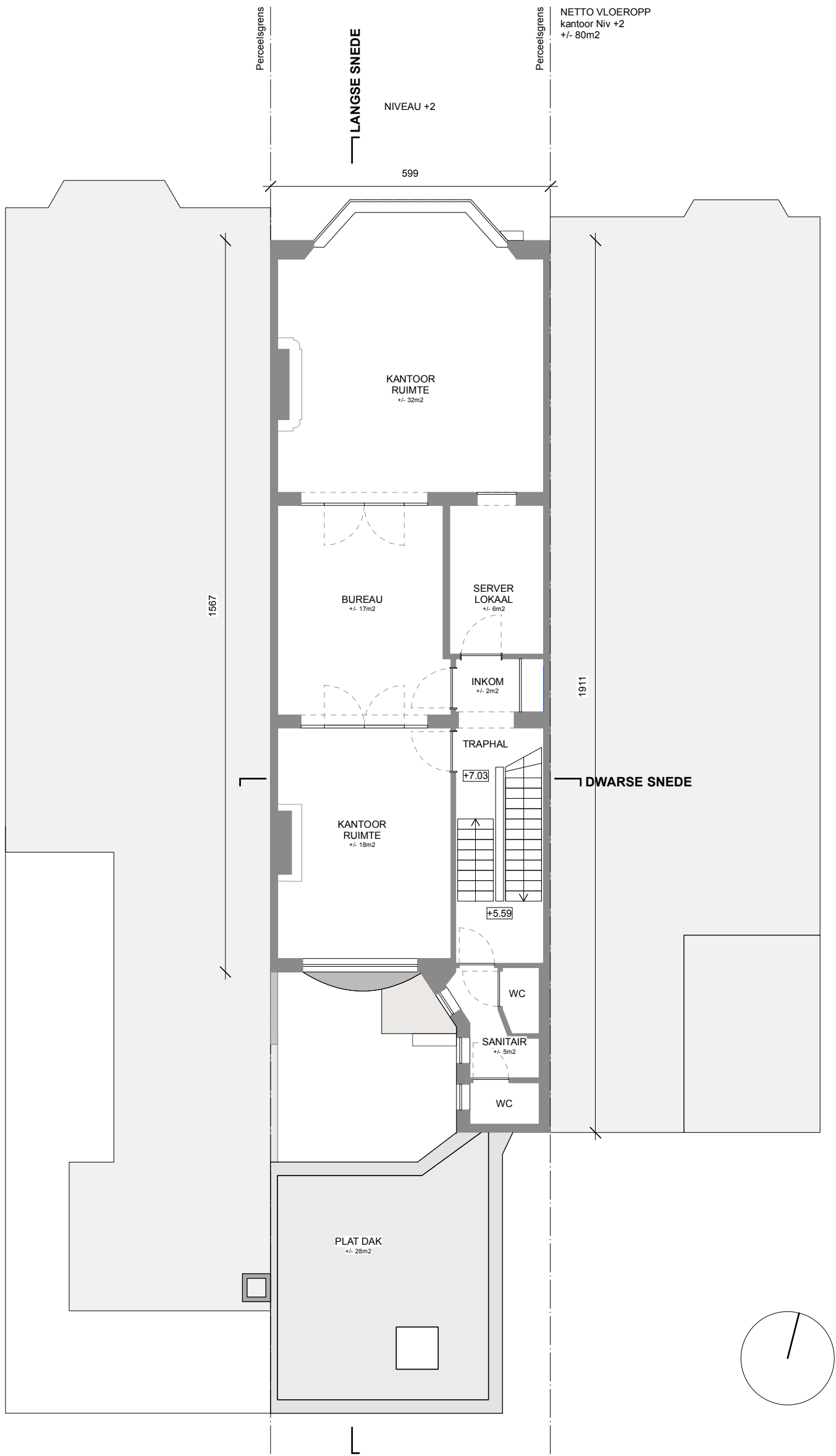
PLAN NIV+2 BESTAANDE TOESTAND schaal 1/100
