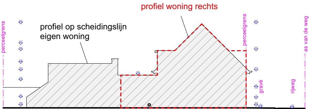
TERREINSNEDE AA' (bestaande)
