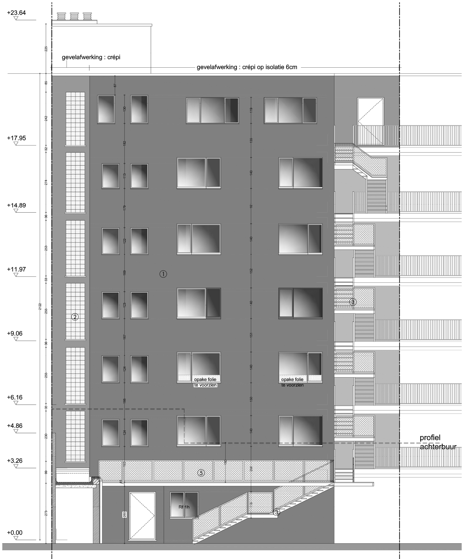
ACHTERGEVEL
