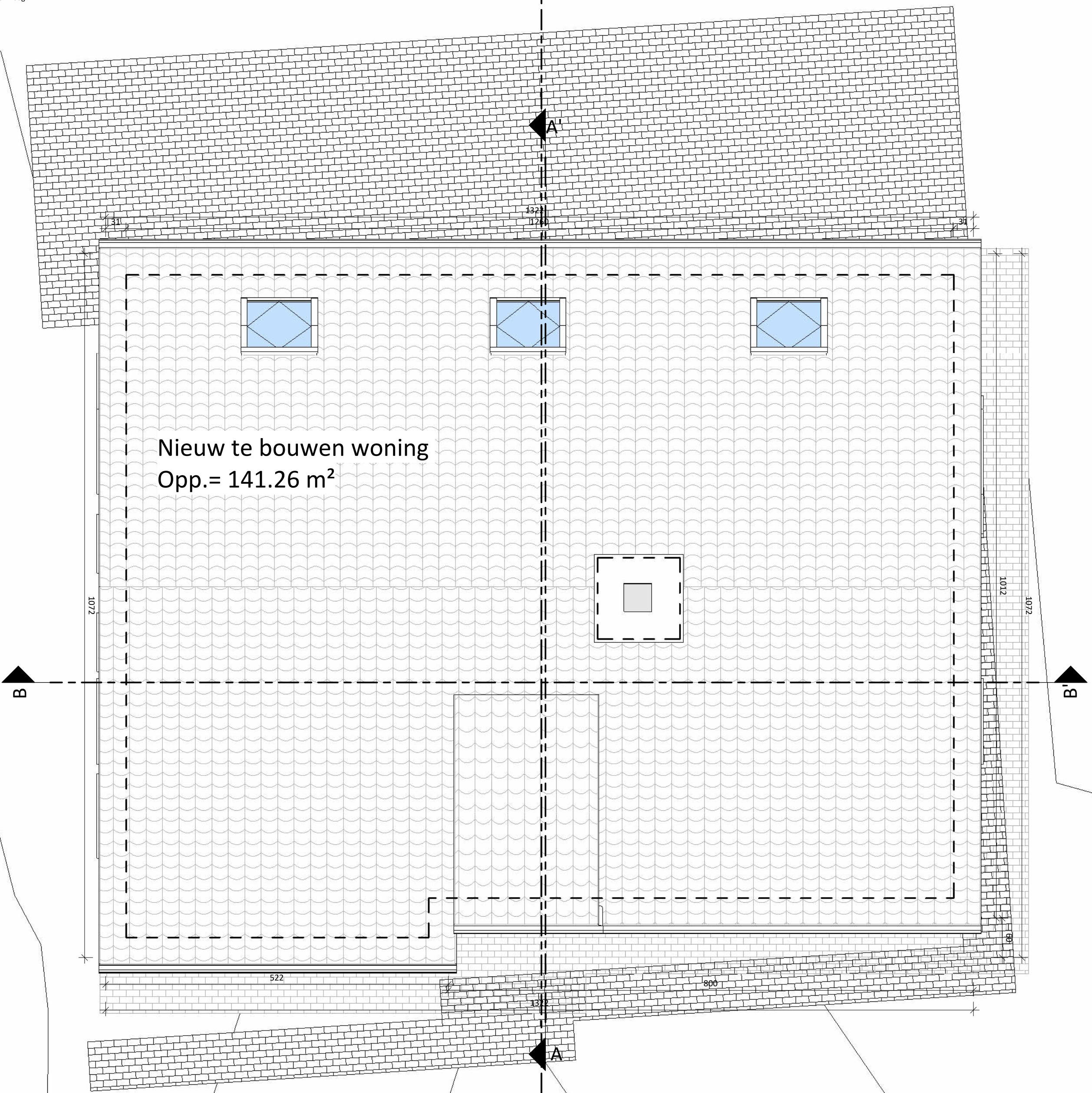
Dakenplan | Nieuwe toestand | 1 : 50
