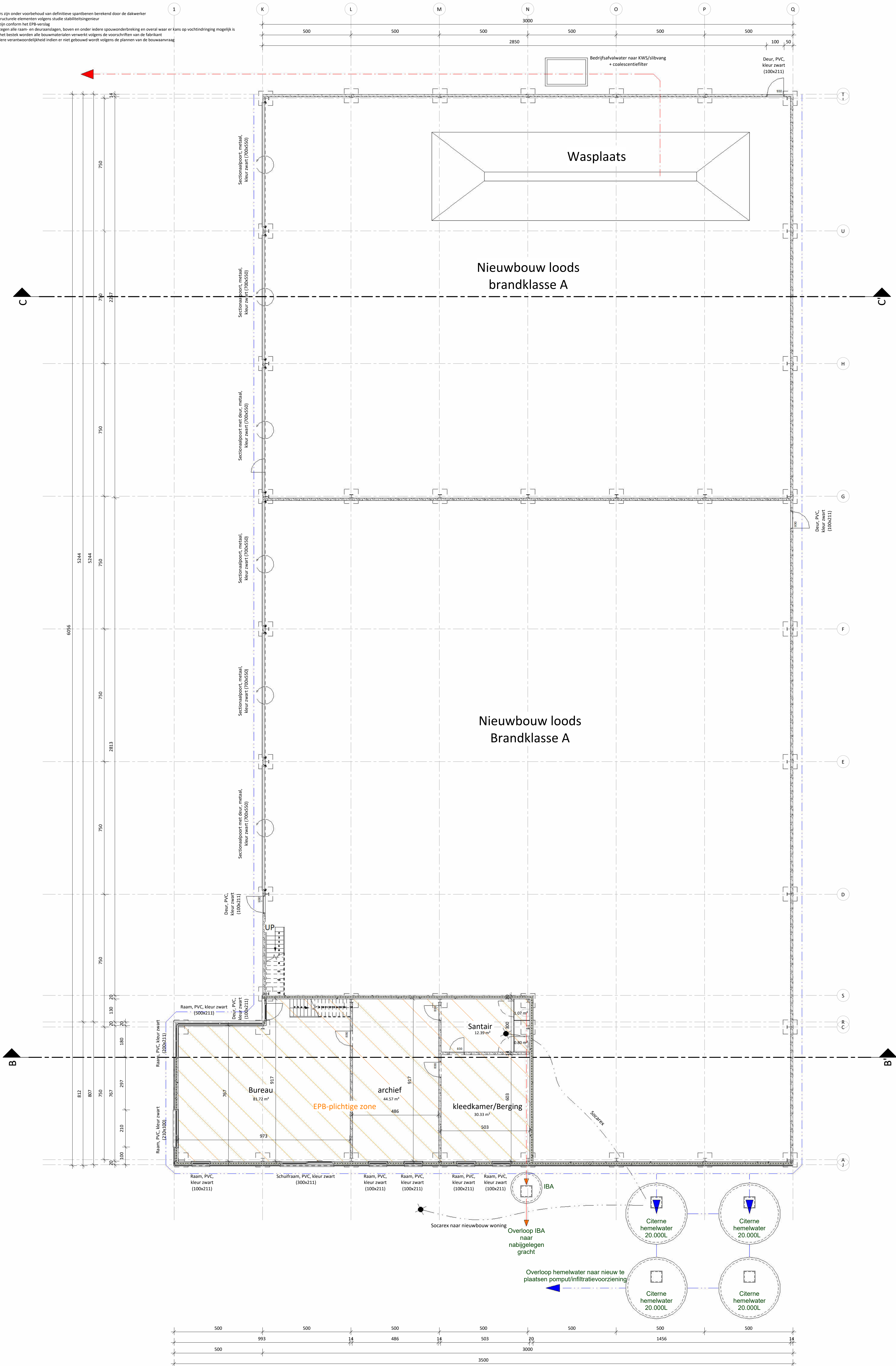
Grondplan gelijkvloers | Nieuwe toestand | 1 : 100
