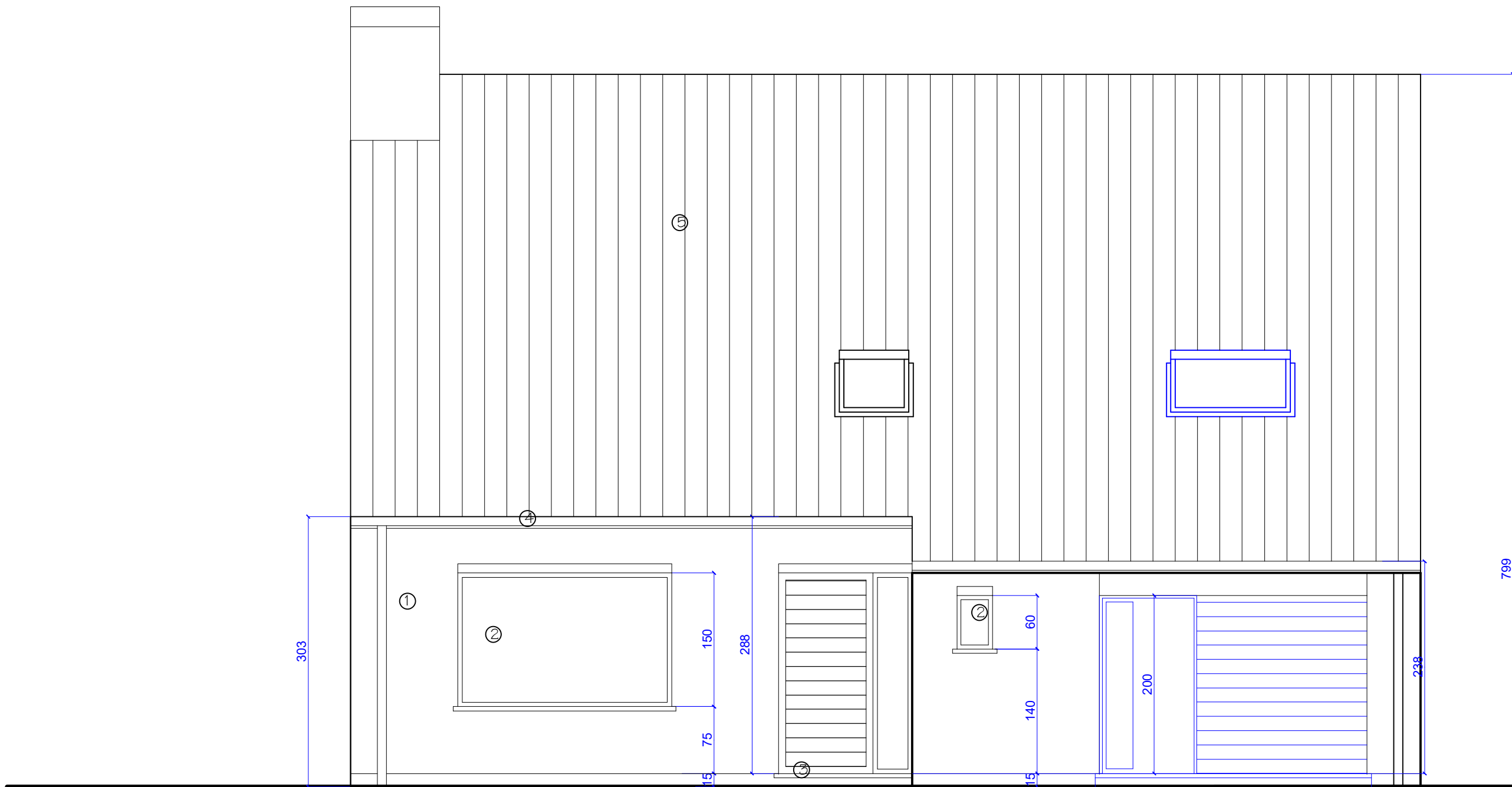
ONTWORPEN VOORGEVEL 1/50
