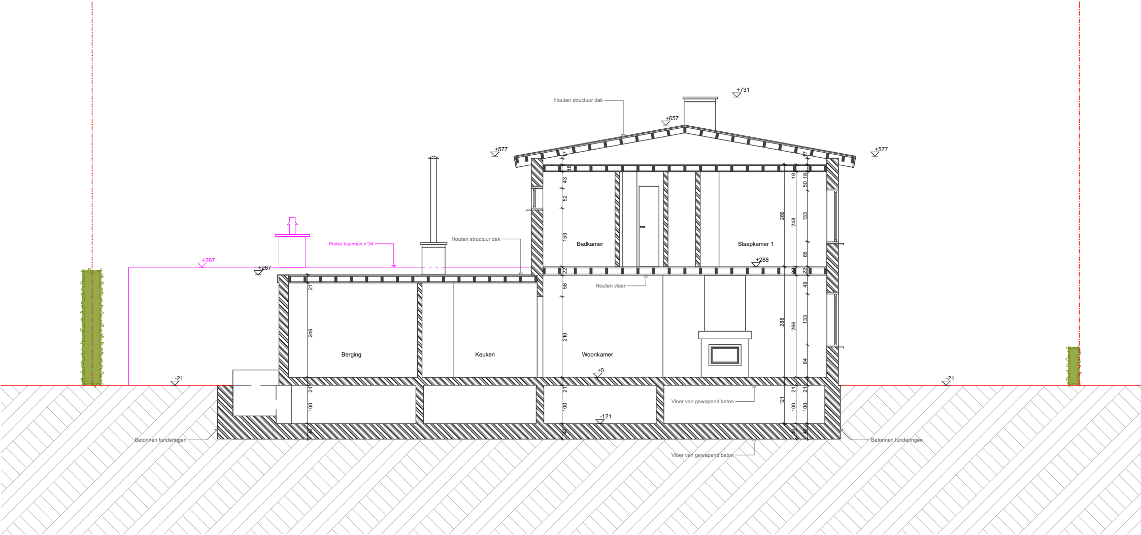
Snede AA
