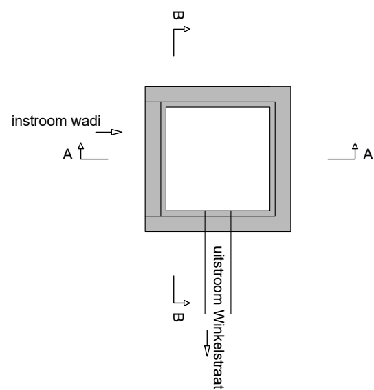
BOVENAANZICHT
