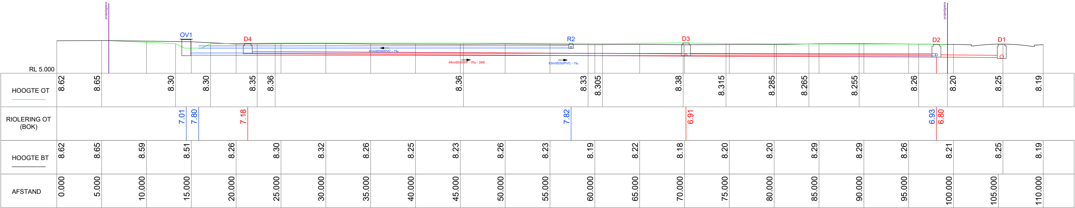
TERREINPROFIEL lengteprofiel A Ch 0.000 to Ch 113.451 SCALES: HORIZONTAL 1:250 VERTICAL 1:250
