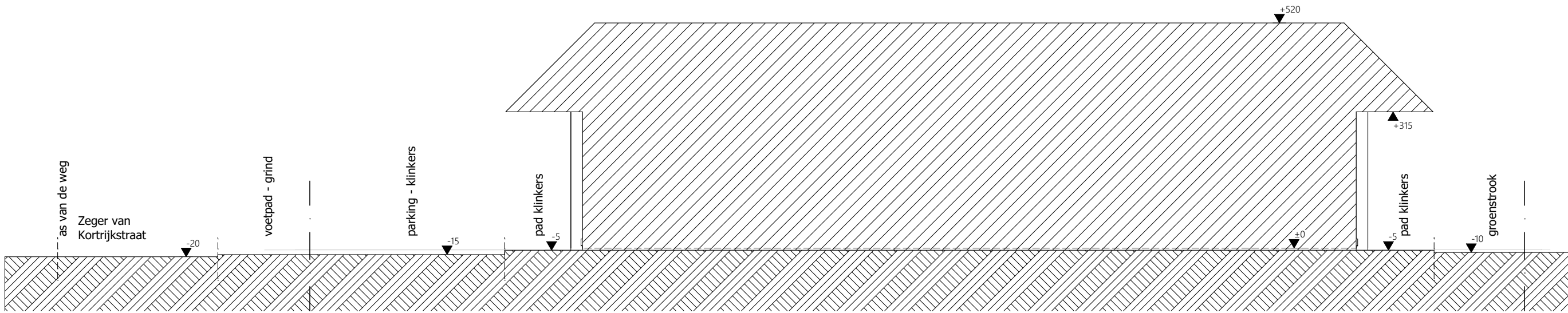
TP Terreinprofiel - bestaande toestand 1:100
