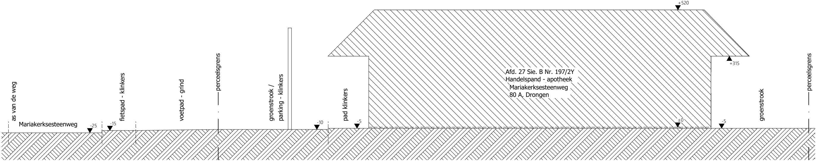
TP Terreinprofiel B - bestaande toestand 1:100
