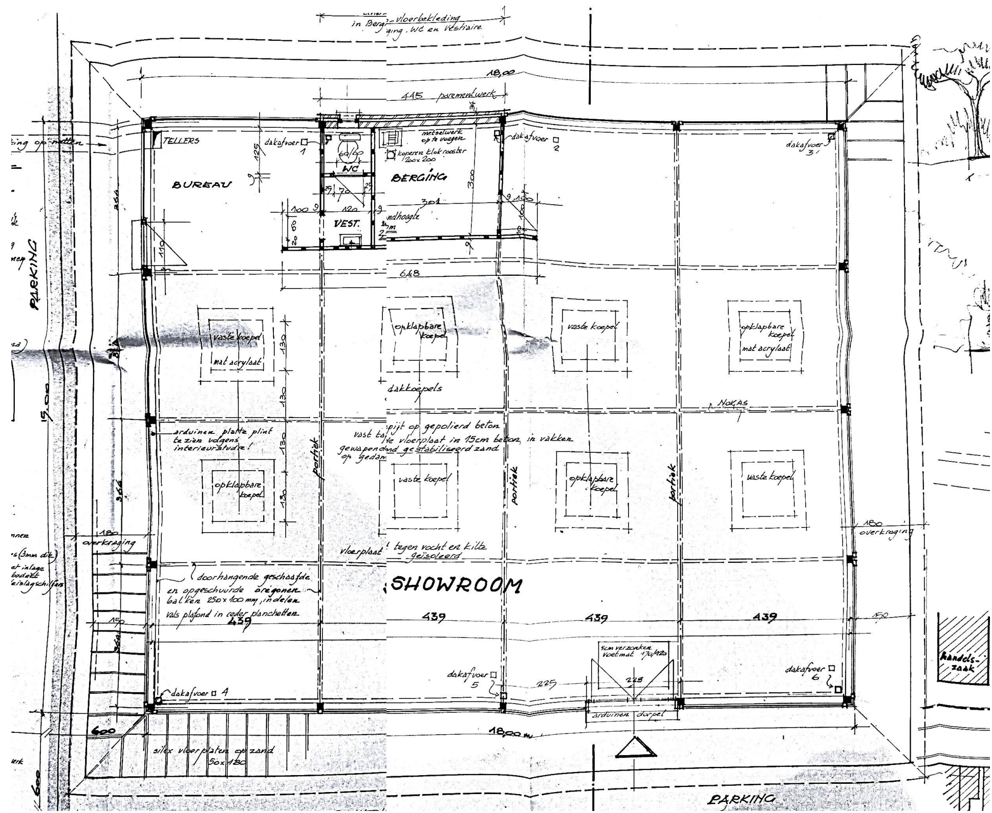
-2. Grondplan niveau 0 - vergunde toestand 1:100
