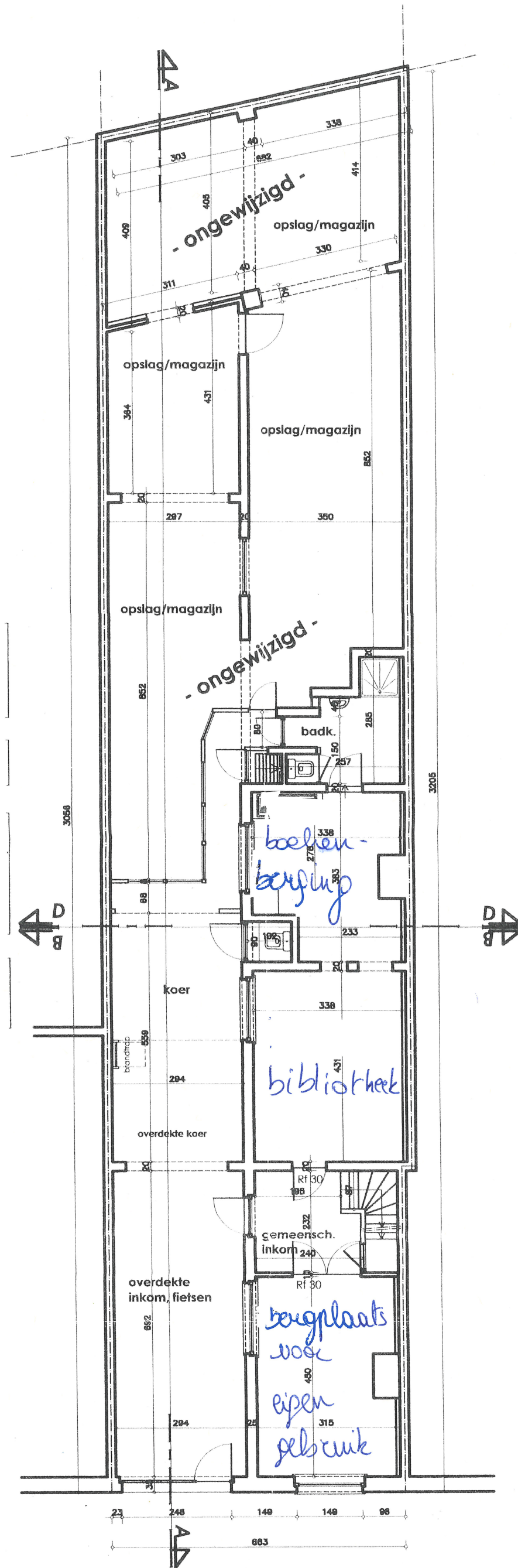
grondplan NT = BT
