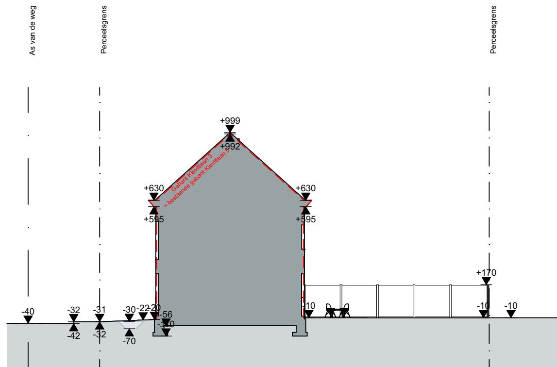
Terreinprofiel NT, 1:200
