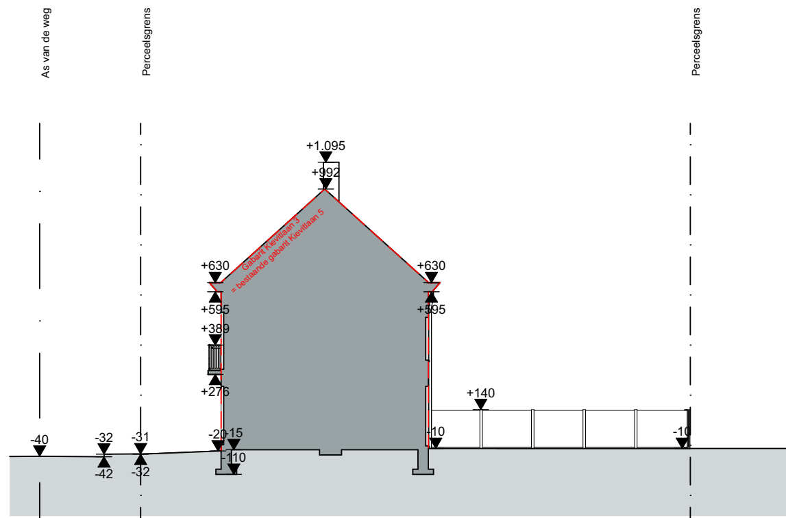
Terreinprofiel BT, 1:200
