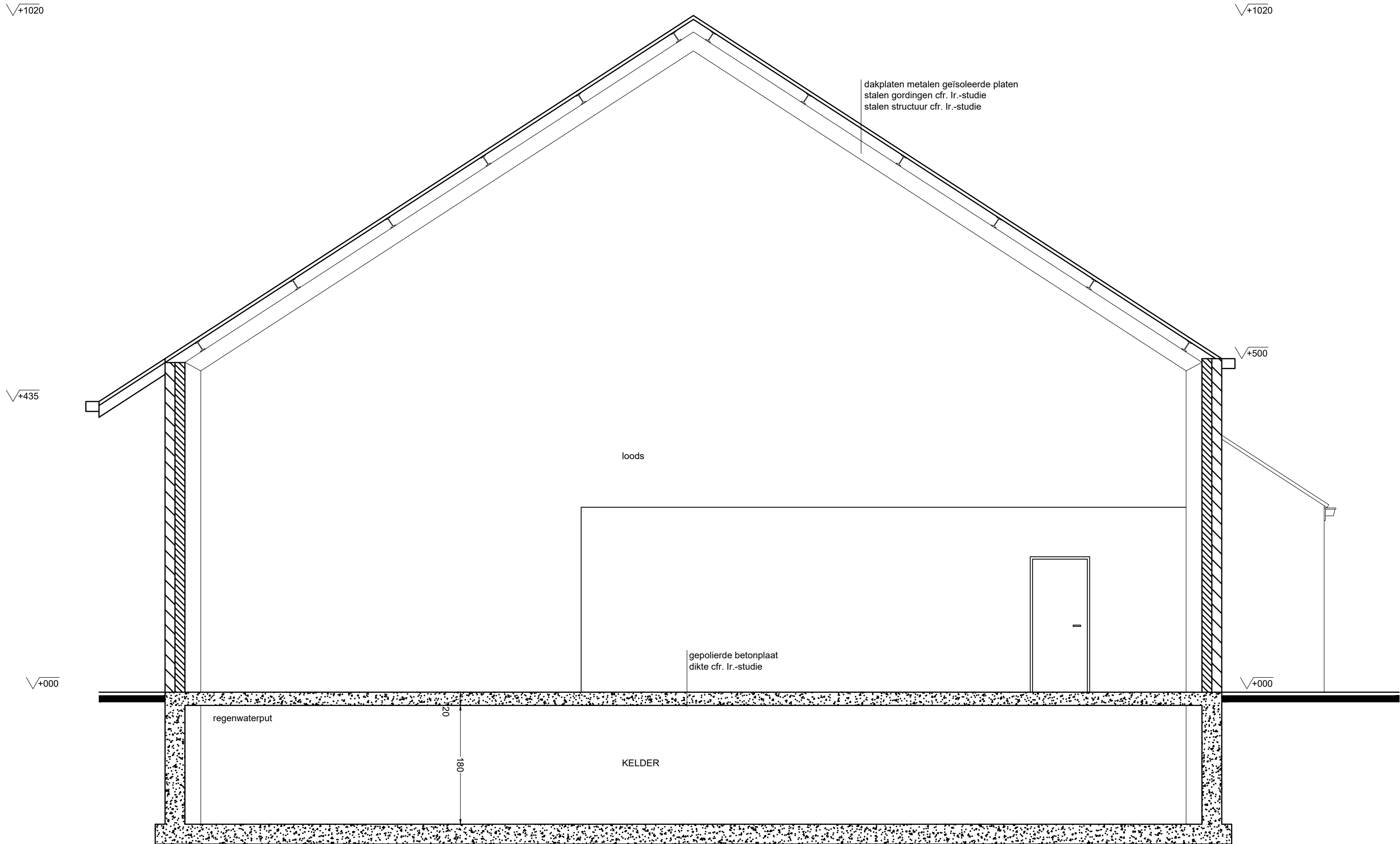
DOORSNEDE BB LOODS nieuwe toestand
