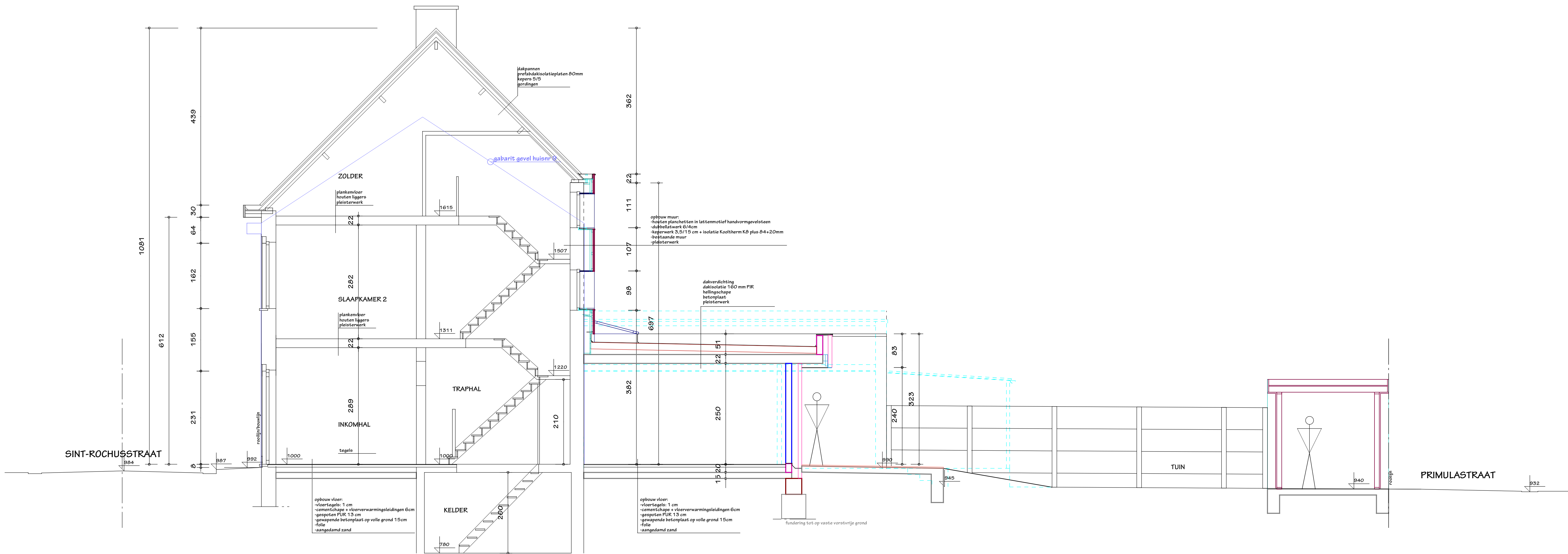
DOORSNEDE BB
