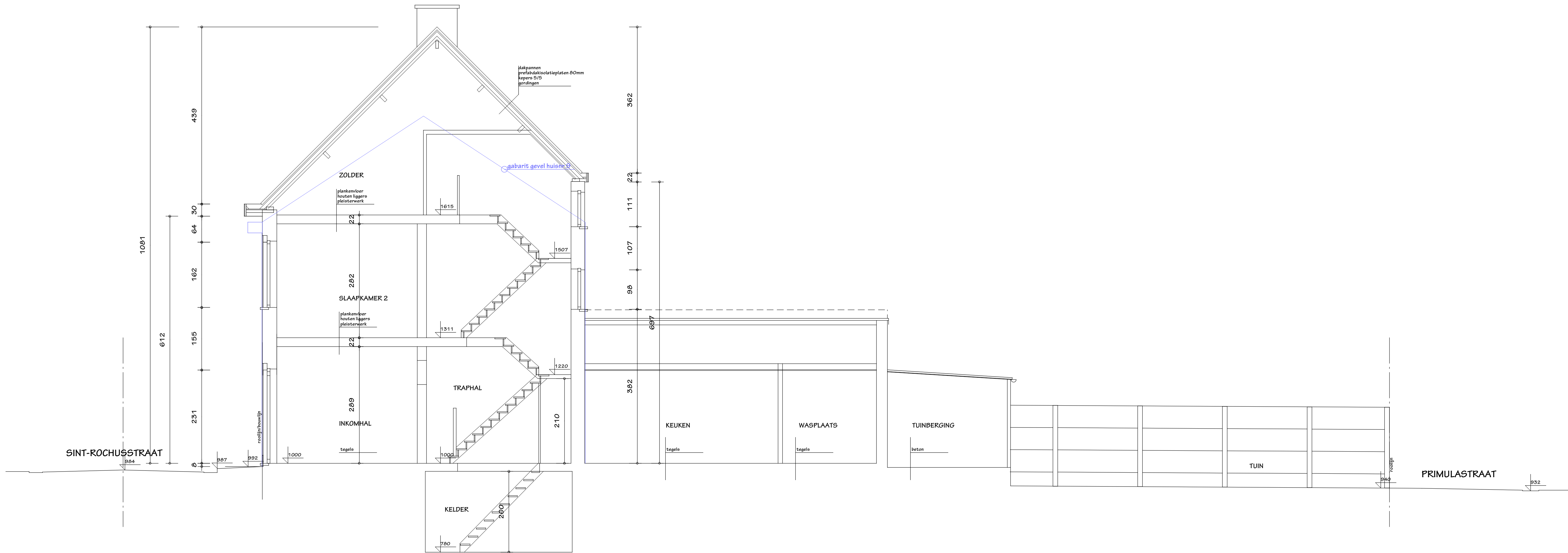
DOORSNEDE BB
