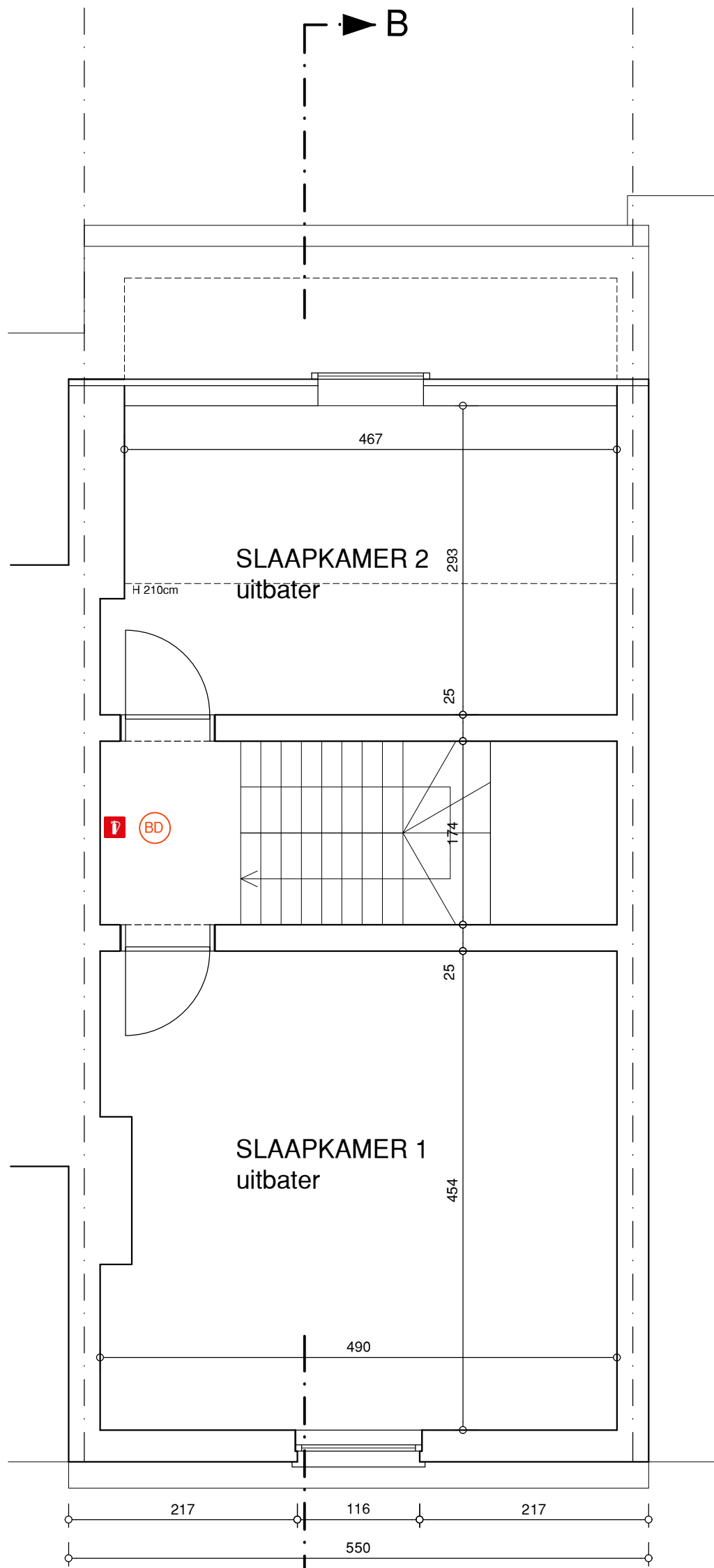
VERDIEPING 3
