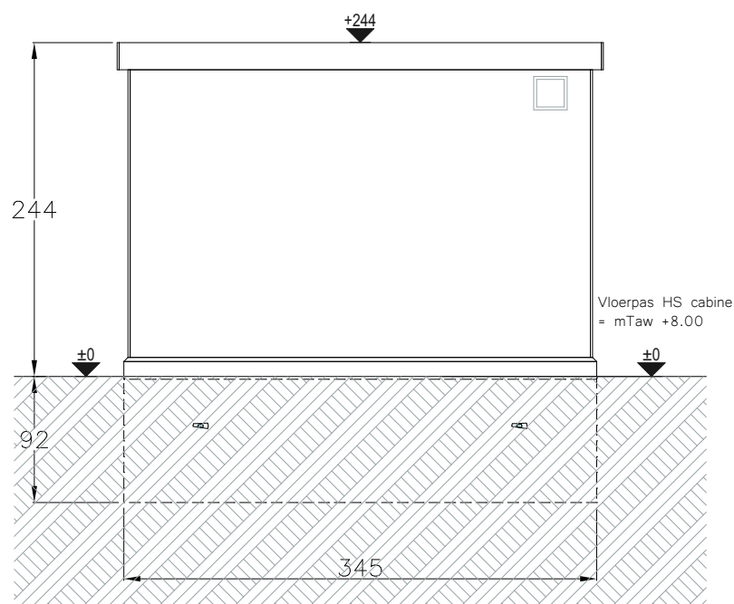
Aanzicht voor
