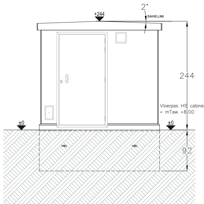
Aanzicht rechts
