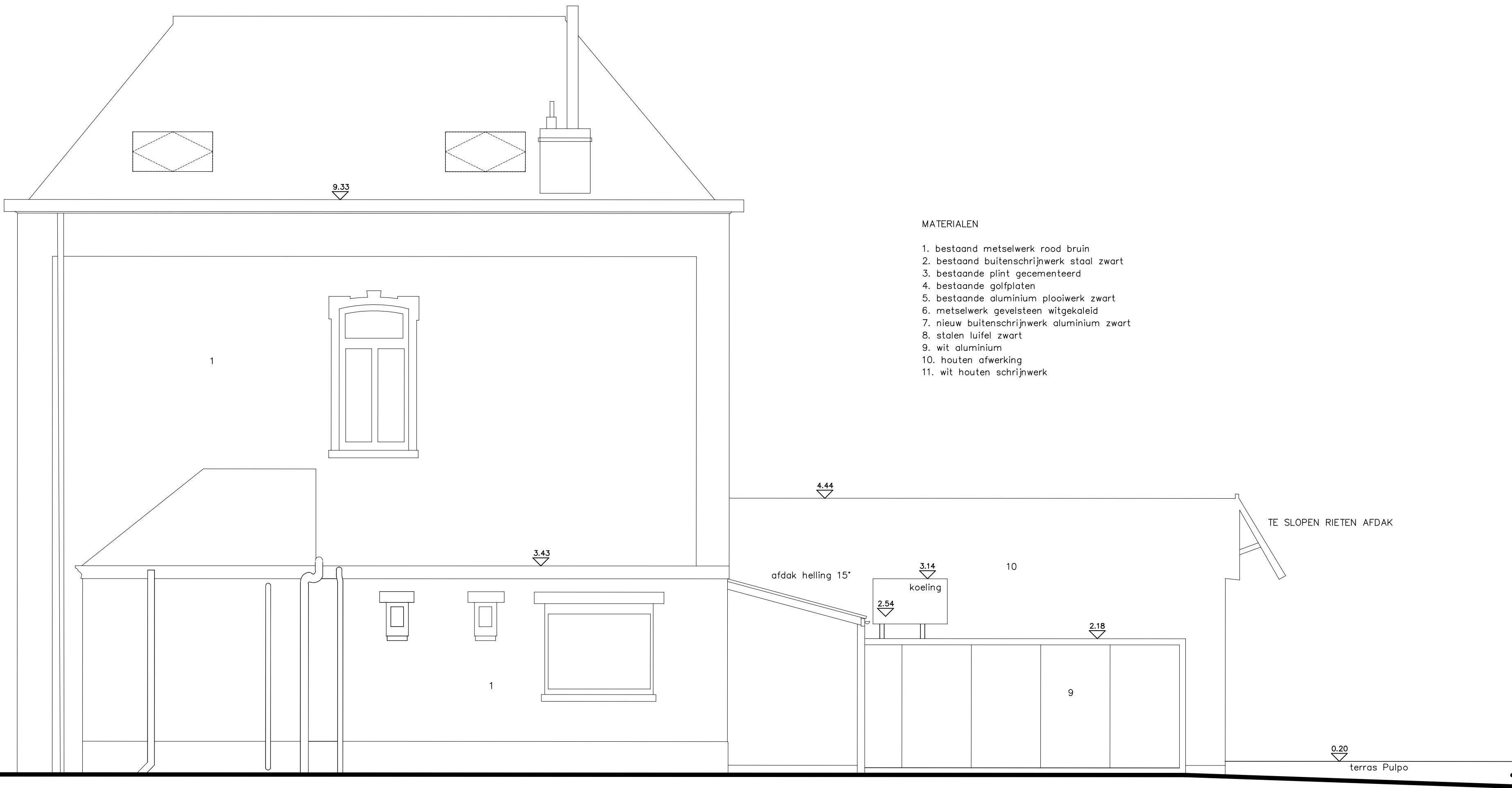
Gevel west (parkzijde) bestaande toestand
