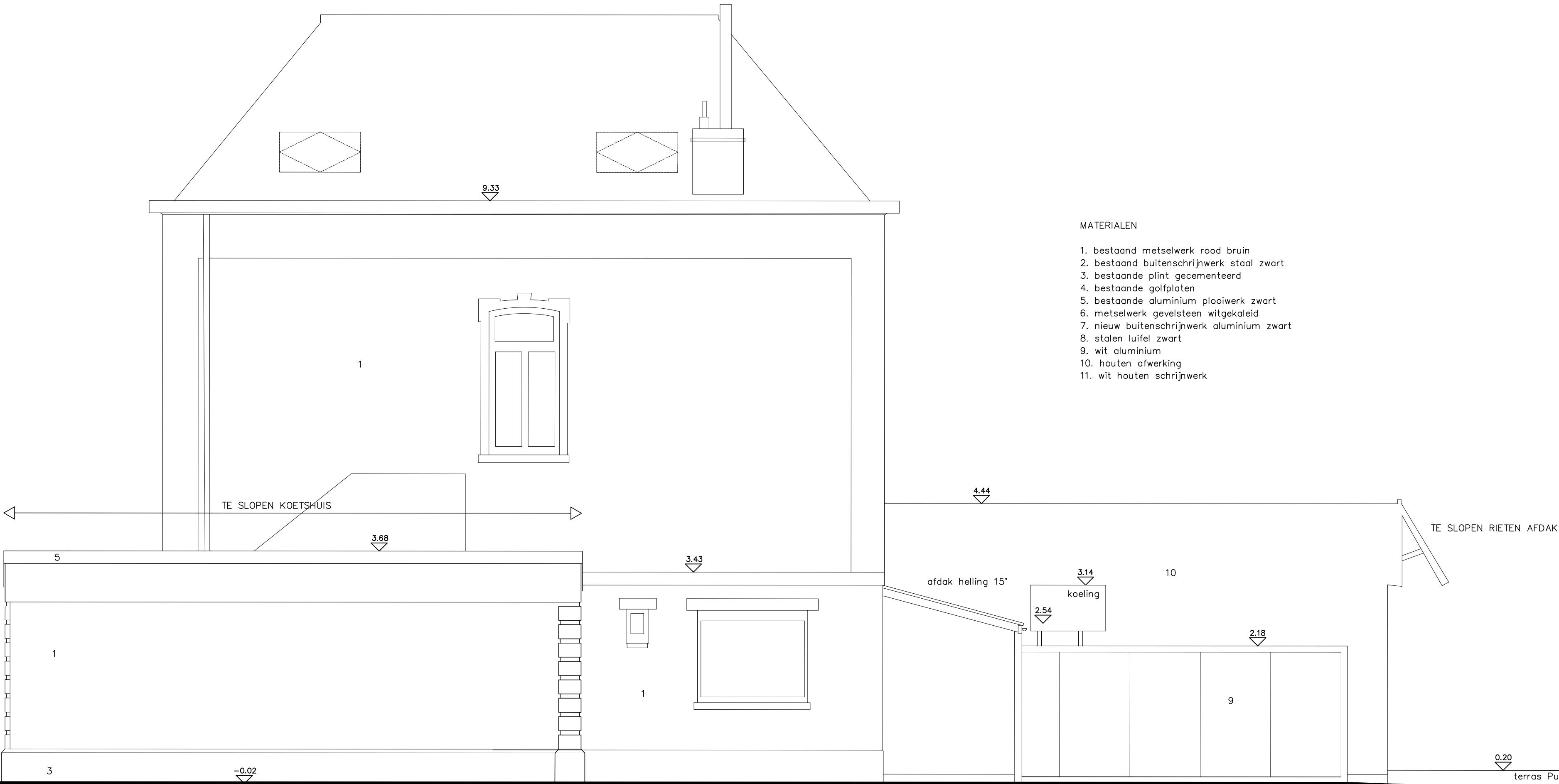
Gevel west (parkzijde) bestaande toestand
